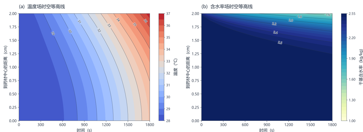
图4 预热阶段外层先升温、先失水，中心含水率在 30 min 内变化很小。左、右图分别为温度与干基含水率的时空等值线，纵轴为距中心的径向位置；等值线数值的单位分别为 ^{\circ}\text{C} 和 \text{kg/kg} 。
