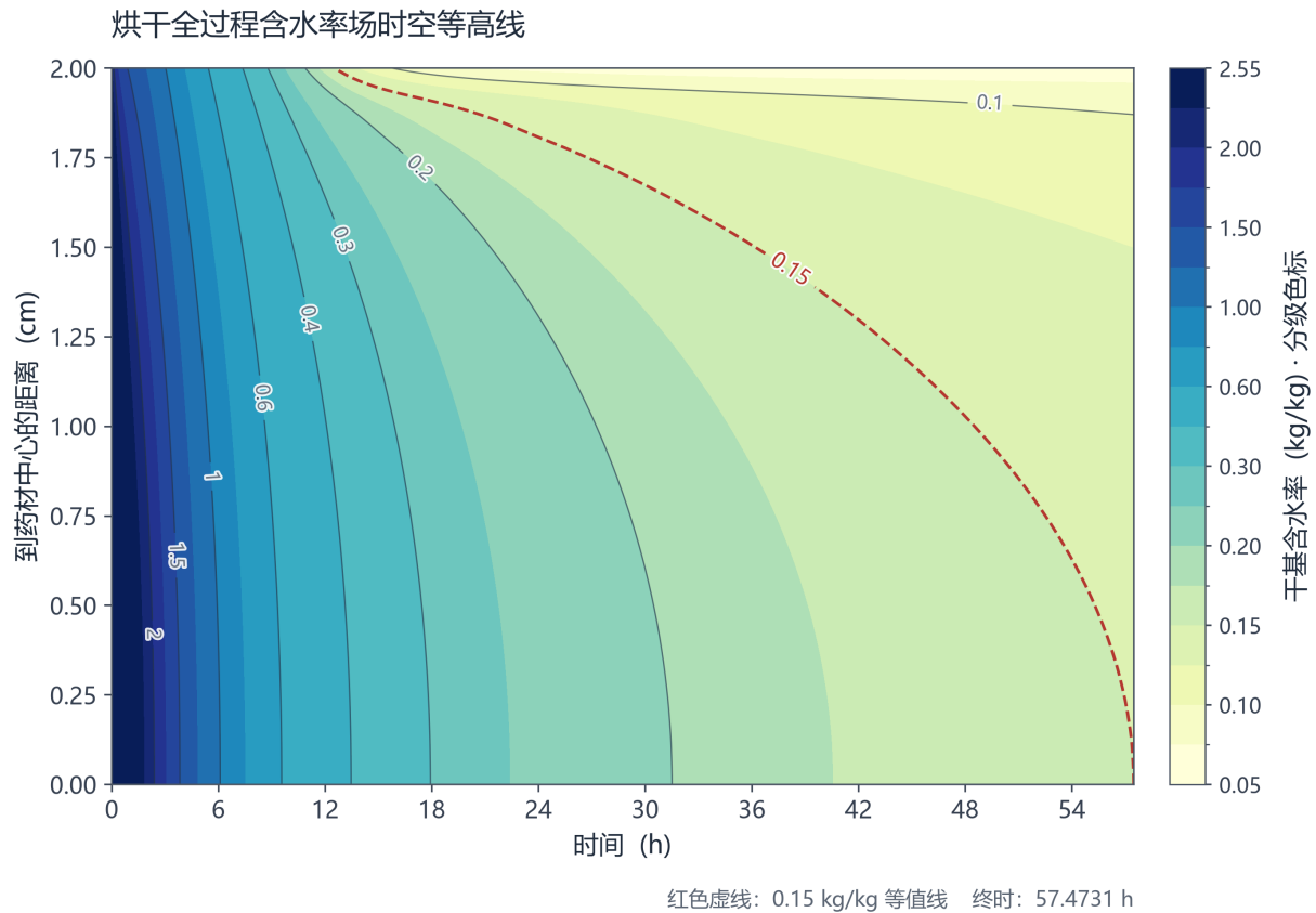
图 7 表层先达标，未达标区域随时间向中心收缩。红色虚线为 C = 0.15 \text{ kg/kg} 等值线，其到达中心对应临界时刻；图示止于稍晚的严格达标报告时刻 57.4731 h。填色采用非等距分级，以区分低含水率阶段的变化。
