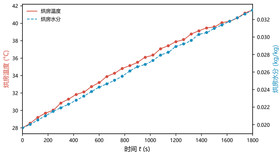
图 1 前 30 min 烘房温度和水分量随时间变化，曲线由附件 1 观测插值得到。
