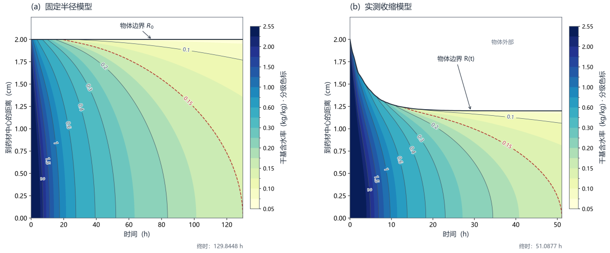
图 11 同一附录 4 物性下，收缩组比固定半径组更早达标。左、右图分别为固定半径组与实测半径驱动收缩组的计算含水率场，时间轴范围不同，采用相同的非等距分级色标；红色虚线为 C = 0.15 \text{ kg/kg} 等值线，黑线为药材边界。图中终时分别为两组严格达标报告时刻 129.8448 h 和 51.0877 h。
