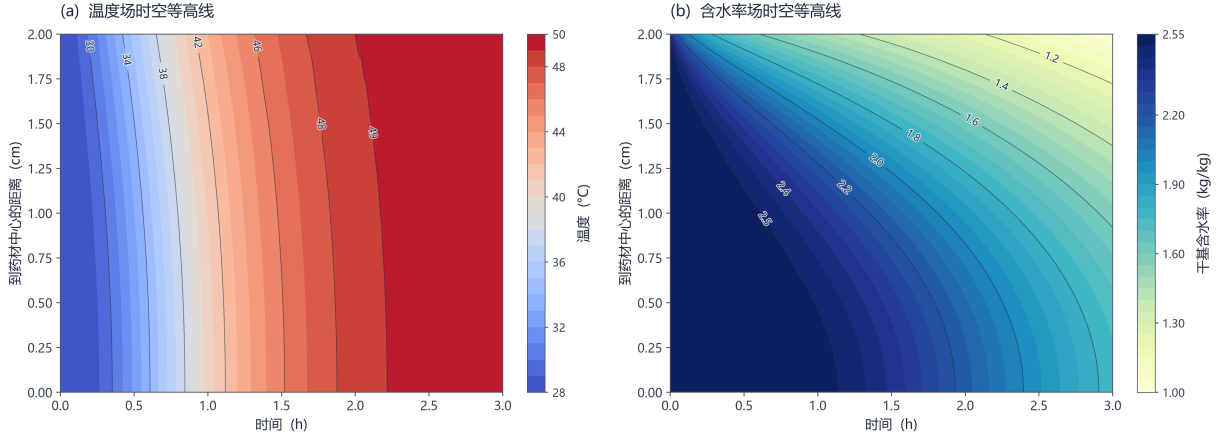
图 5 前 3 h 温度逐渐接近烘房水平，水分仍保持中心高、表面低的径向差异。左、右图分别为变物性模型的温度与干基含水率时空等值线，等值线数值的单位分别为 ^{\circ}\text{C} 和 \text{kg/kg} 。
