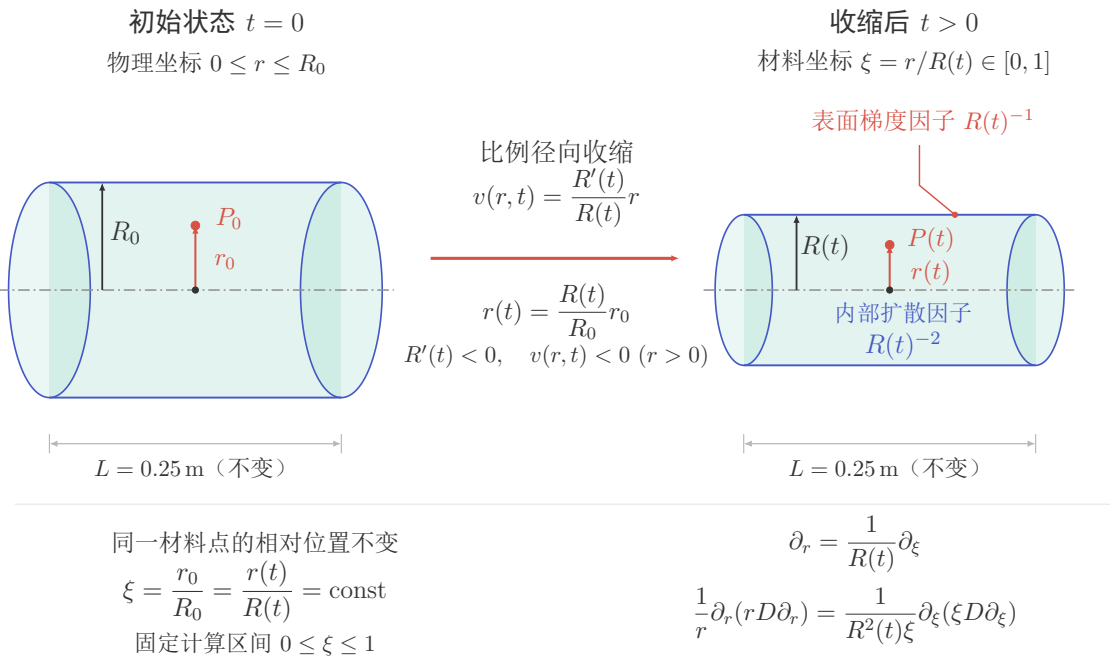
图 9 比例径向收缩与材料坐标示意。坐标变换使表面梯度与内部扩散分别带有 R(t)^{-1} 和 R(t)^{-2} 几何因子；收缩比例、材料点位置及长径比仅作示意，不对应特定实测时刻。
