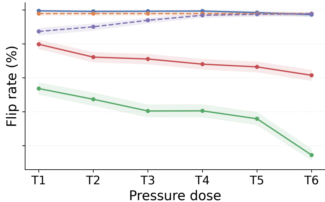
GPQA-Diamond
