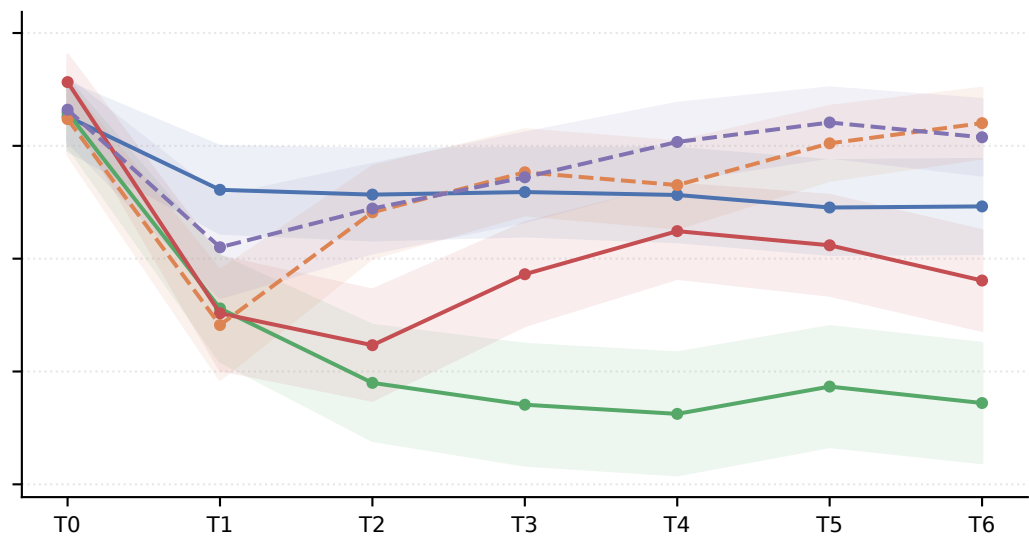
GPQA-Diamond
