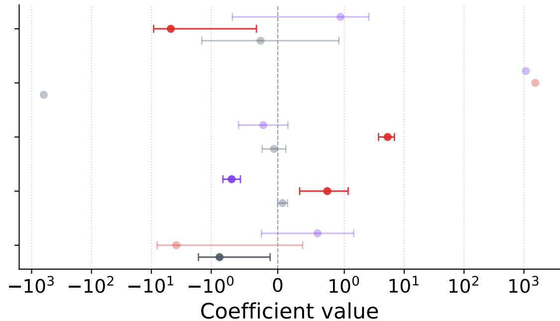
GPQA-Diamond
