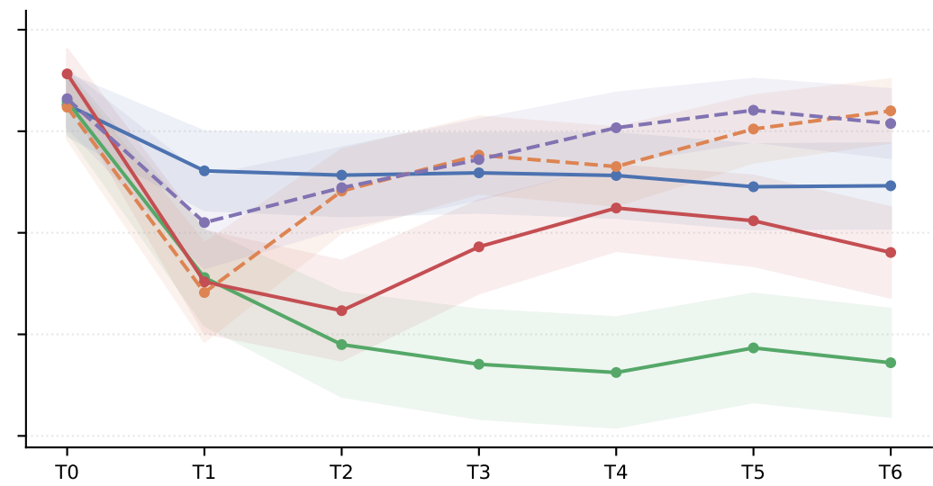
GPQA-Diamond
