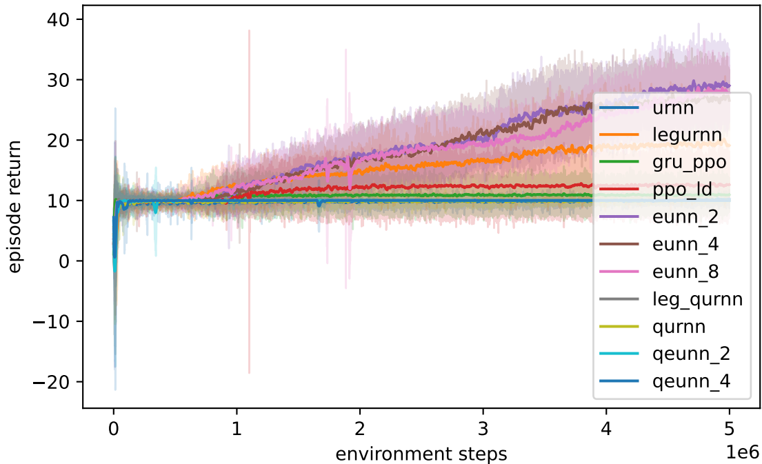
rocksample_11_11
