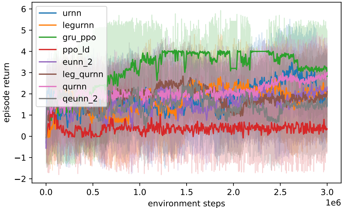
tmaze_75
