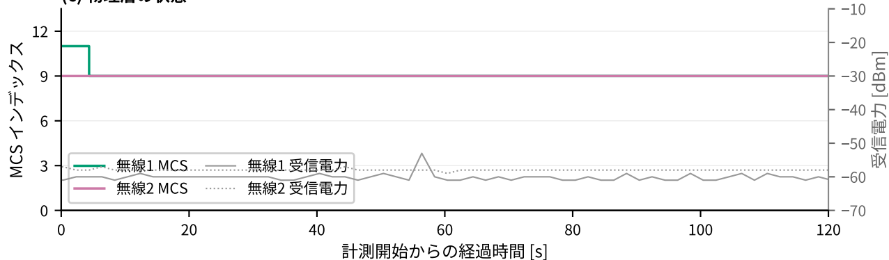
(c) 物理層の状態
