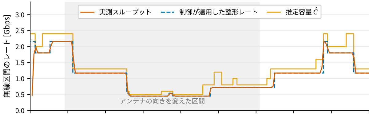
(b) 受信ノードのスループット
