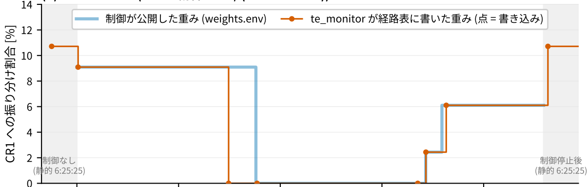
(c) 重みの変更から経路表への反映まで (区間は時刻分解能 1 s による幅)
