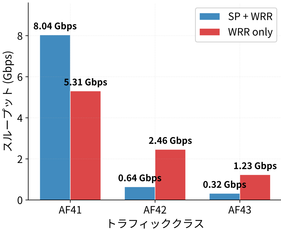
(a) クラス別スループット
