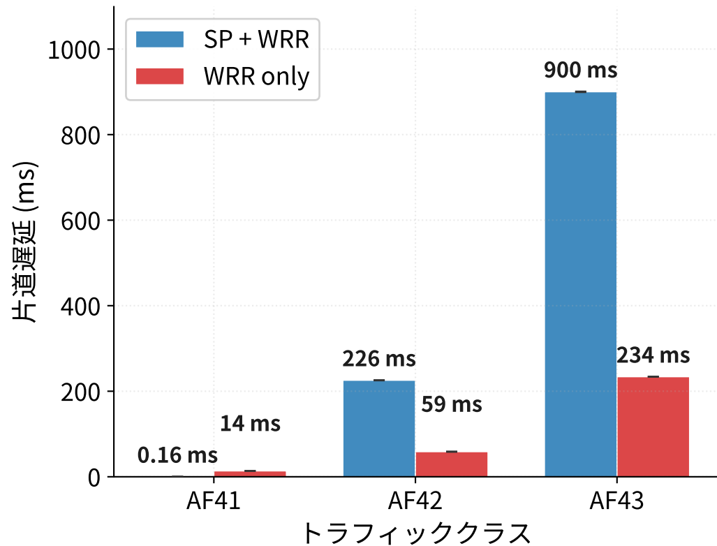
(b) クラス別片道遅延 (OWD)
