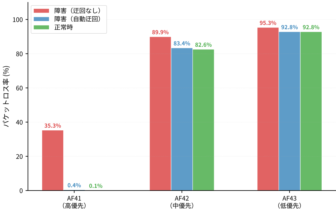
UDP パケットロス率 (iperf3 実測, 60 s 平均)
