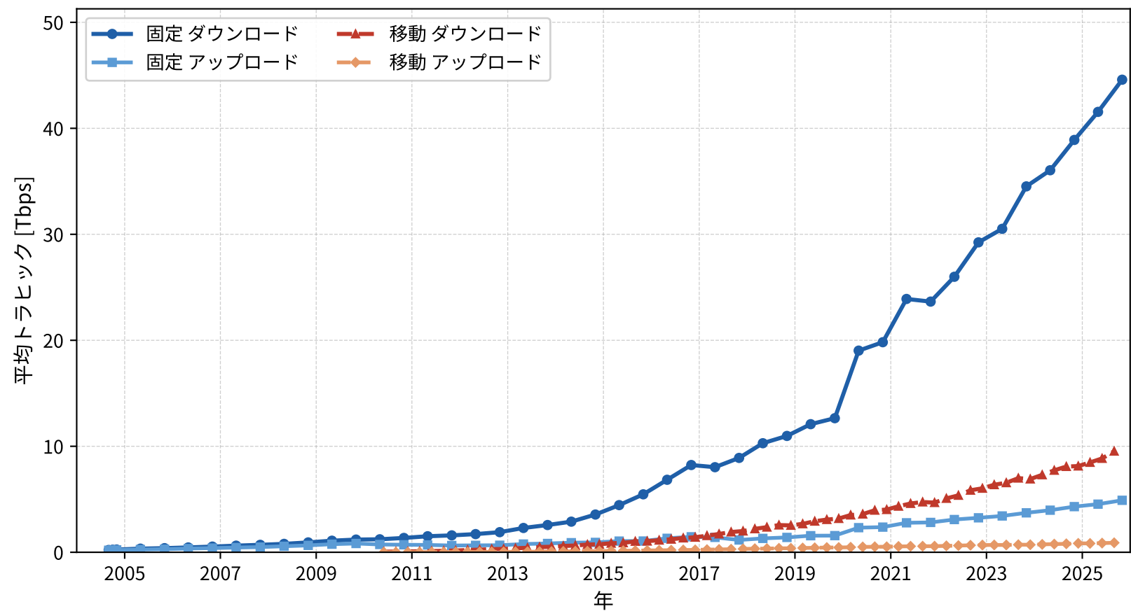
我が国の固定通信・移動通信トラヒックの推移（総務省）
