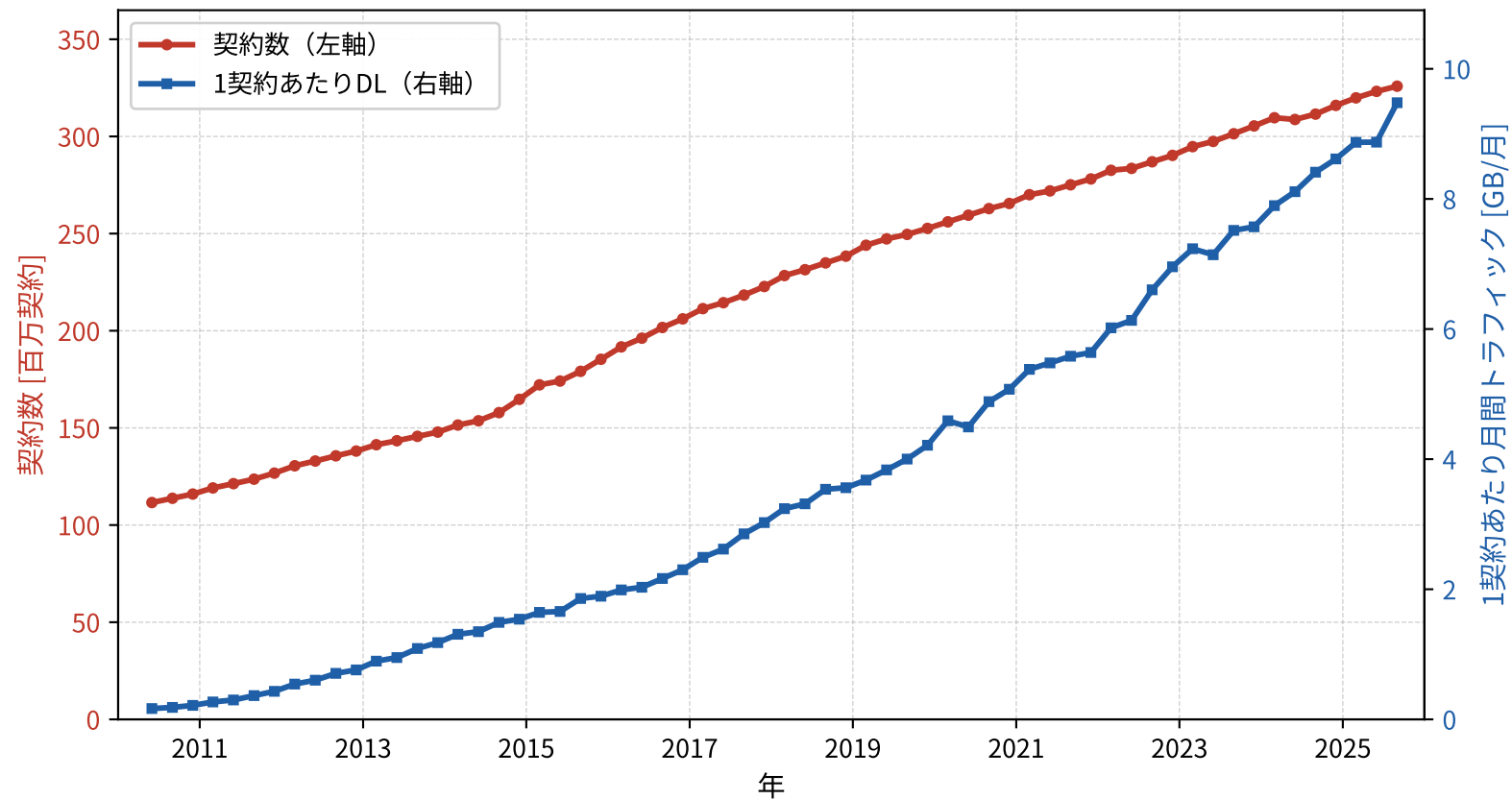
移動通信：契約数と1契約あたり月間トラフィック（総務省）
