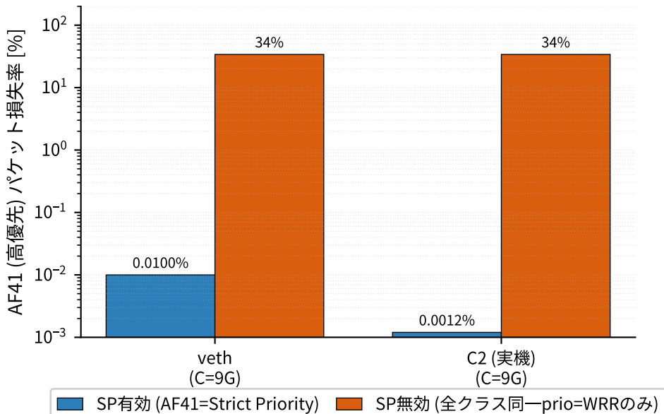
AF41 損失率: Strict Priority の有無による比較 (normalシナリオ)
