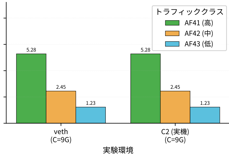
SP無効 (WRR quantum比 4:2:1 のみ)
