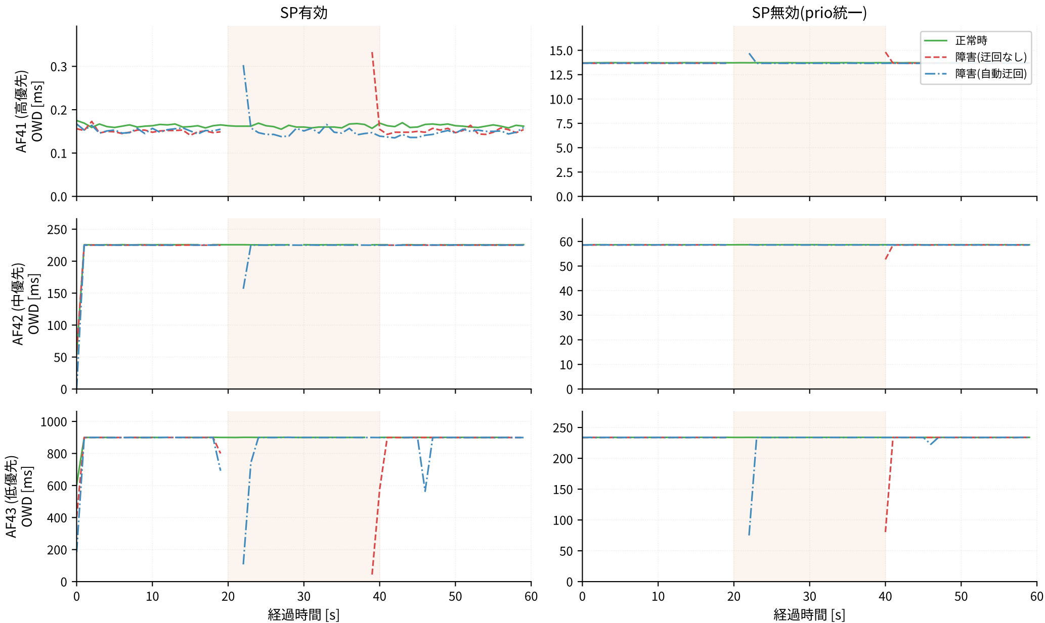
シナリオ別 片道遅延OWD時系列 — SP有効 vs SP無効 の統合比較 (C2 (実機) (C=9G), 障害区間 t=20~40s 網掛け, 1秒中央値)
