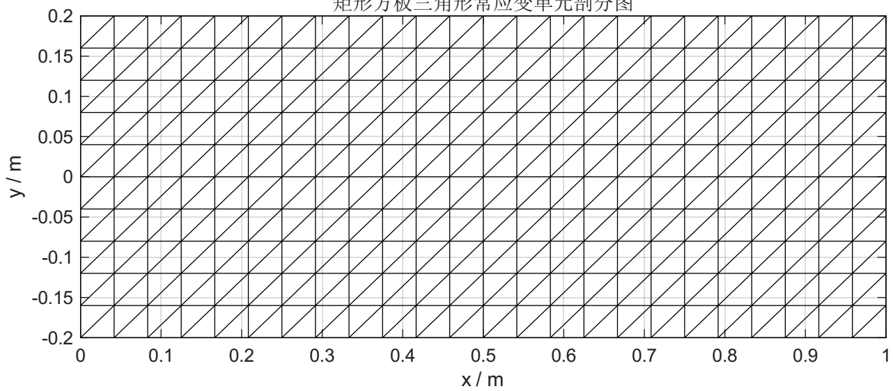
矩形方板三角形常应变单元剖分图
