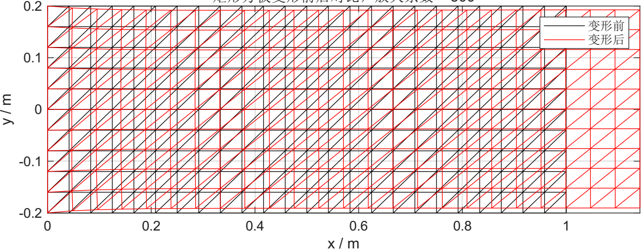
矩形方板变形前后对比，放大系数 = 300
