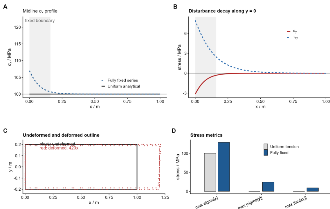
图 4 边界条件对中线应力、扰动衰减、变形轮廓和峰值指标的影响。A, y = 0 上的 \sigma_x 曲线; B, \sigma_y 与 \tau_{xy} 衰减曲线; C, 变形前后轮廓对比, 变形放大 420 倍; D, 两种边界条件下最大 \sigma_x 、最大 |\sigma_y| 和最大 |\tau_{xy}| 对比。
