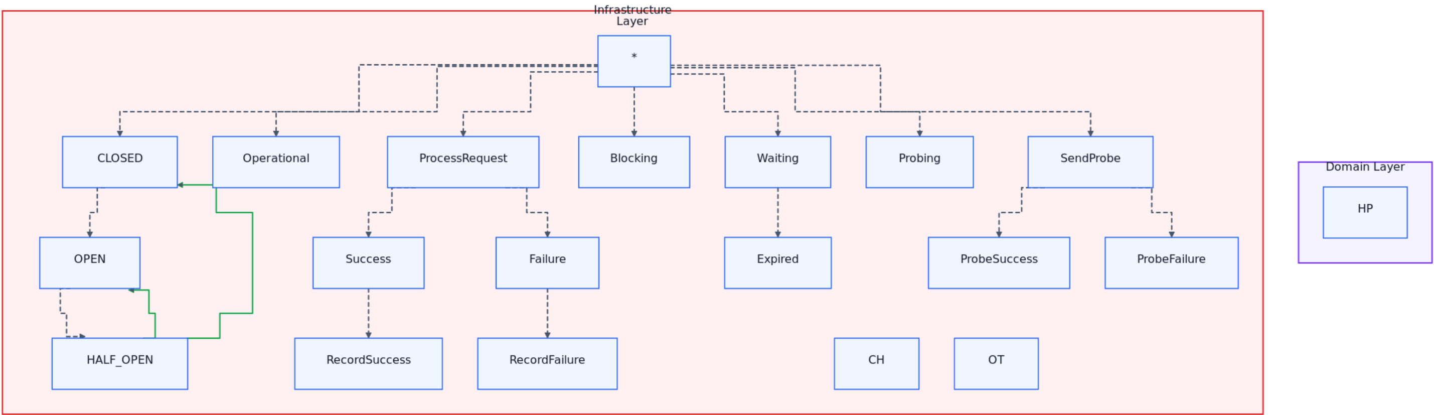
07-circuit-breaker-states-infra
