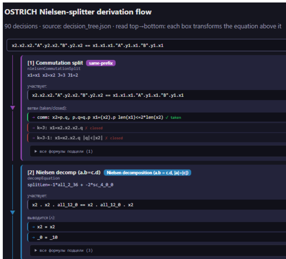
Рисунок 2 — Интерактивный HTML-вид дерева вывода
