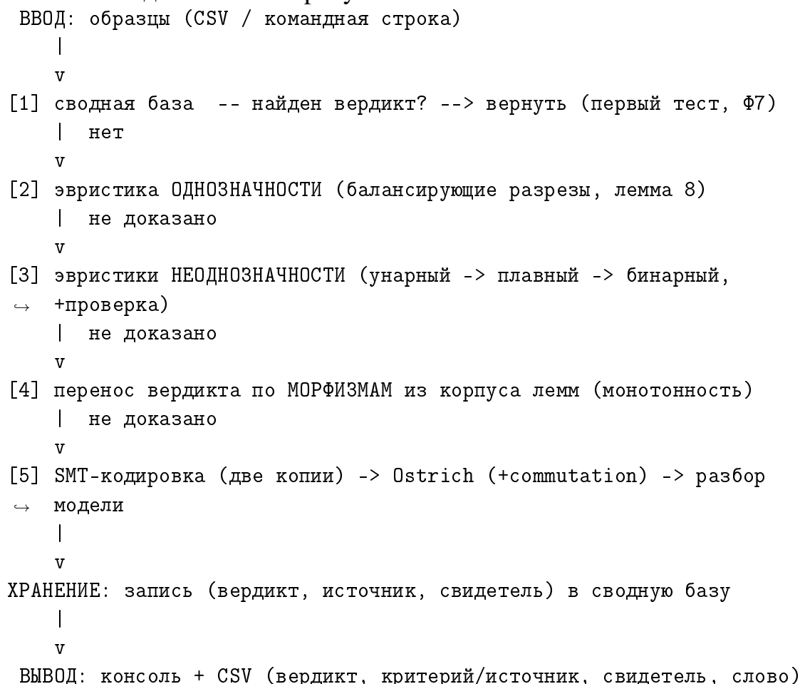
Рисунок 1 — Каркас системы: каскад методов и поток данных
