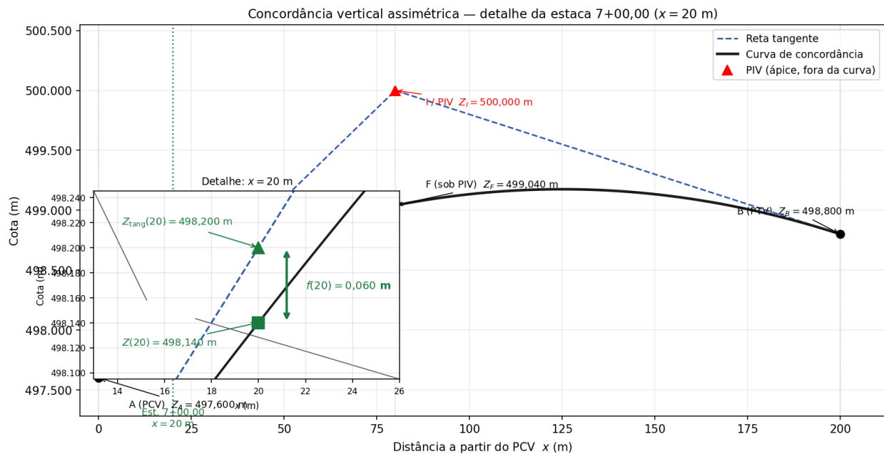
Figura 1: Perfil longitudinal da concordância vertical assimétrica do exemplo. O inseto amplia a região da estaca 7+00,00 ( x = 20 m), mostrando a cota na reta tangente Z_{\text{tang}}(20) , a cota do greide Z(20) e a flecha local f(20) = 0,060 m entre elas.
