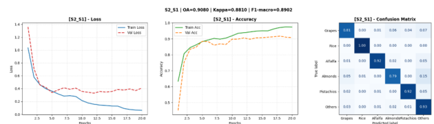
Figure 6.18 – Courbes d'entraînement et validation (MCTNet-v2).
