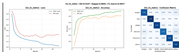
Figure 6.17 – Matrice de confusion de MCTNet-v2 (Californie).
