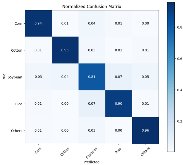
Figure 3.8 – Matrice de confusion du baseline MCTNet sur l’Arkansas.
