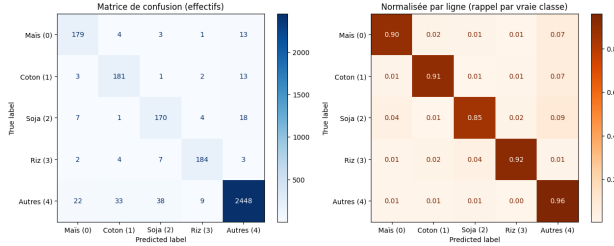
Figure 6.19 – Matrice de confusion du modèle MCTNet-v2 sur l’Arkansas (Partie 3).
