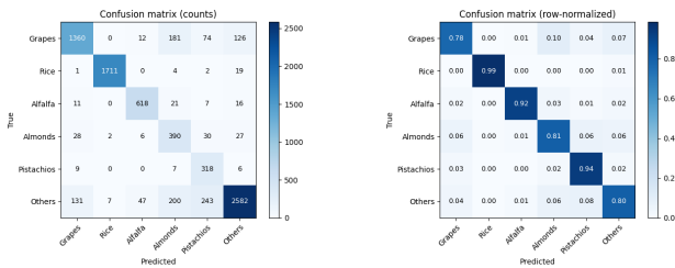
Figure 3.6 – Matrice de confusion du baseline MCTNet sur l'échantillon de test (Californie).
