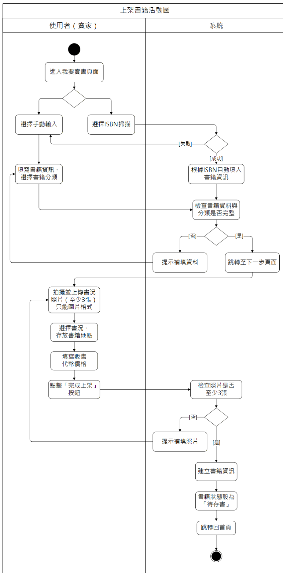
圖 5-3-1 上架書籍之活動圖
