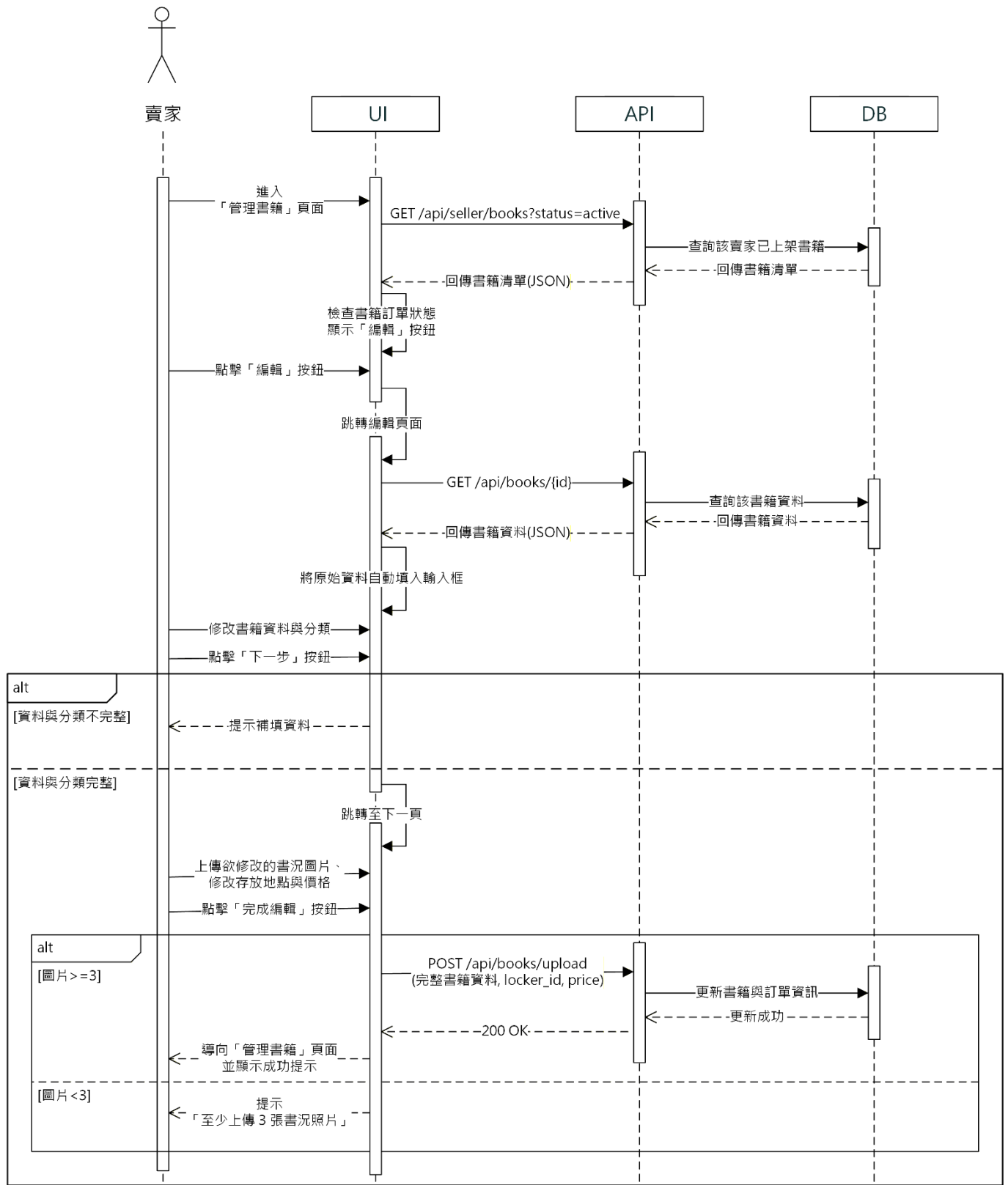
圖 6-1-2 編輯書籍之循序圖
