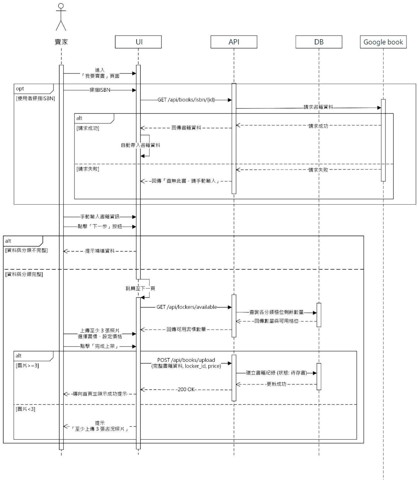
圖 6-1-1 上架書籍之循序圖
