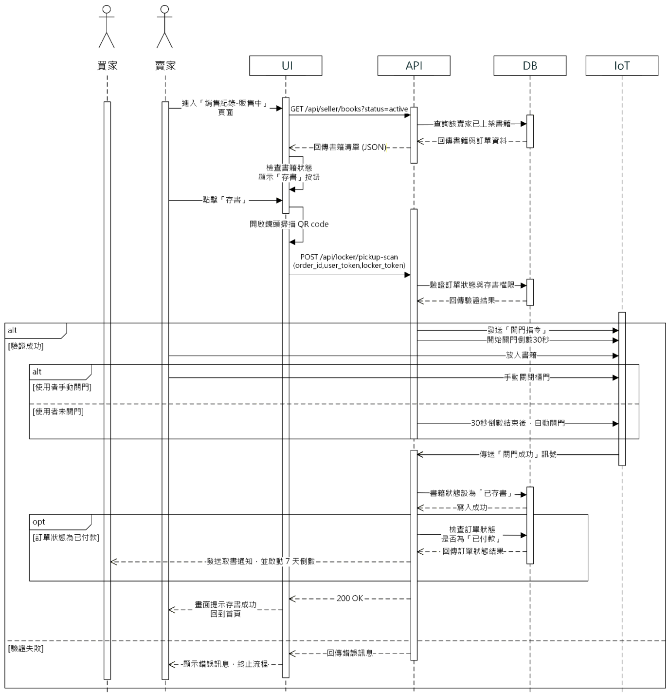
圖 6-1-4 實體書櫃存書之循序圖
