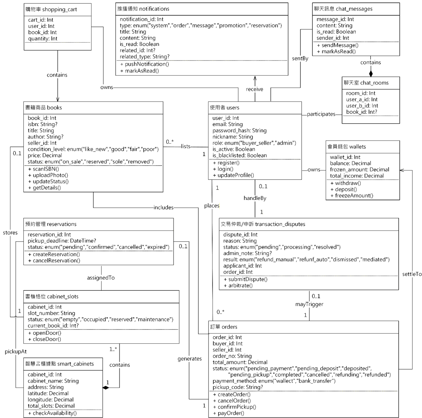
圖 6-2-1 設計類別圖
