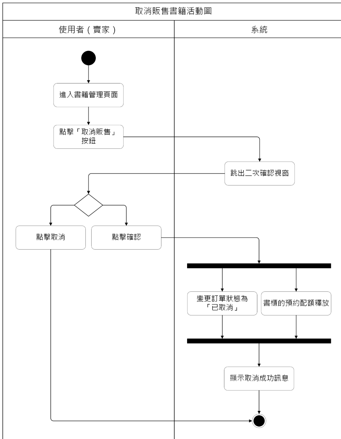
圖 5-3-3 取消販售書籍之活動圖
