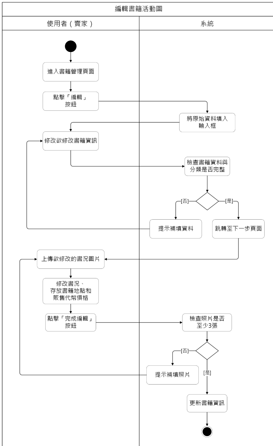
圖 5-3-2 編輯書籍之活動圖
