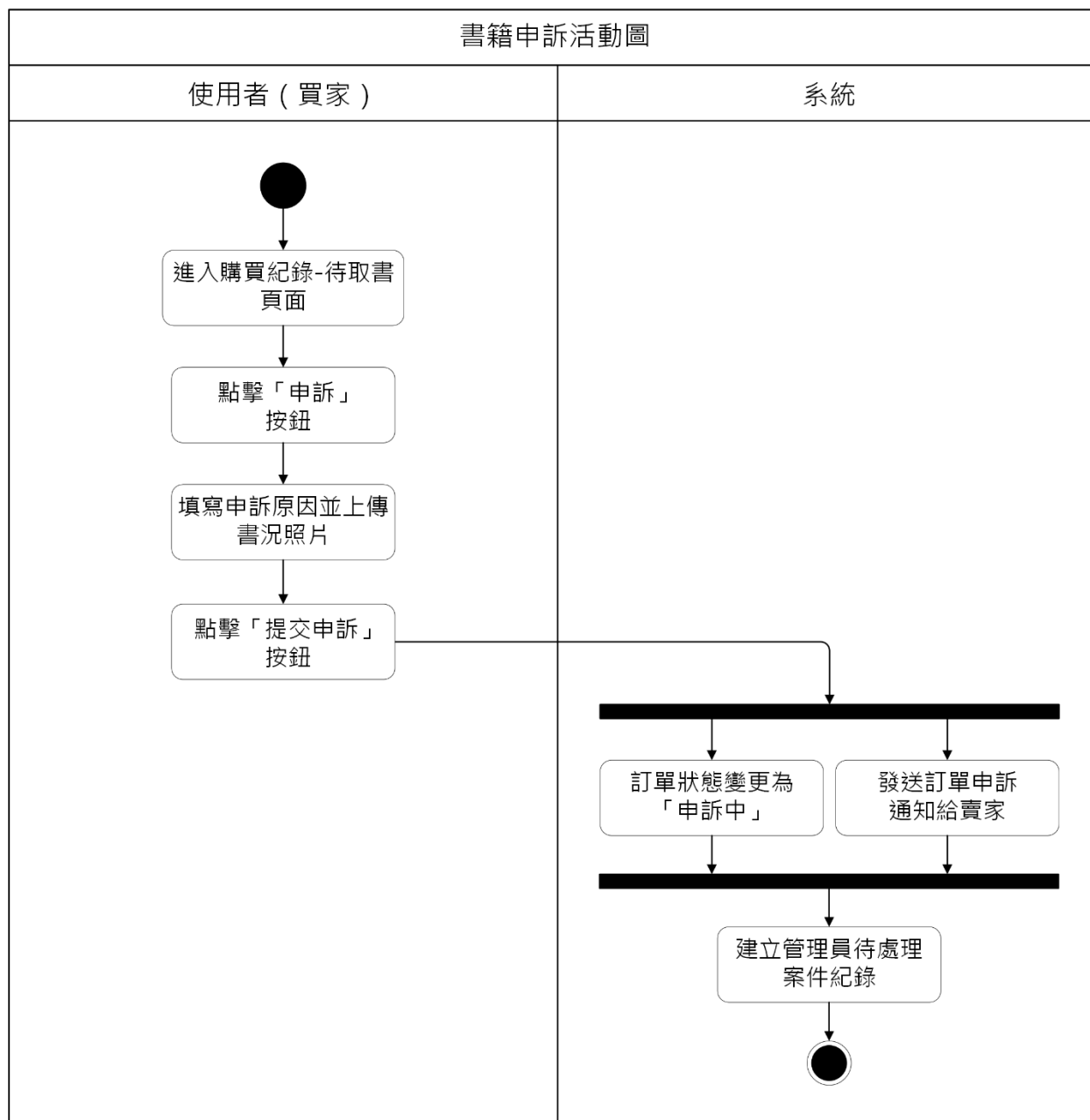
圖 5-3-7 書籍申訴之活動圖
