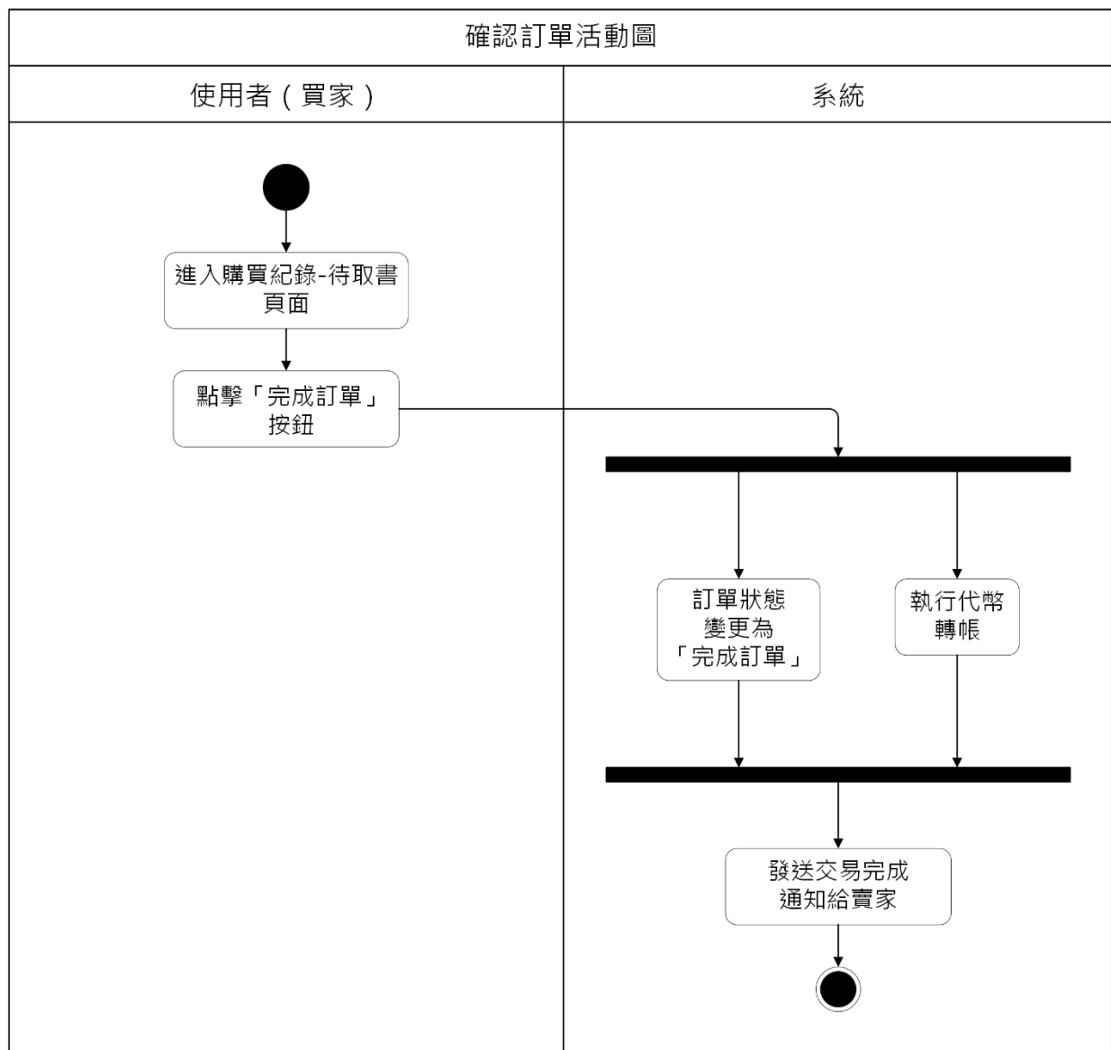
圖 5-3-6 確認訂單之活動圖
