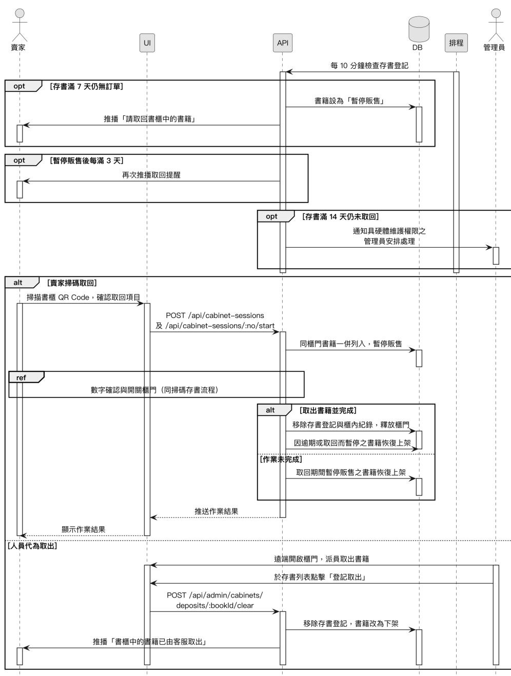
圖 6-1-6 存書逾期暫停與取回之循序圖
