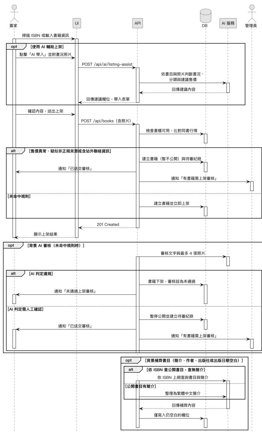
圖 6-1-1 上架書籍之循序圖
