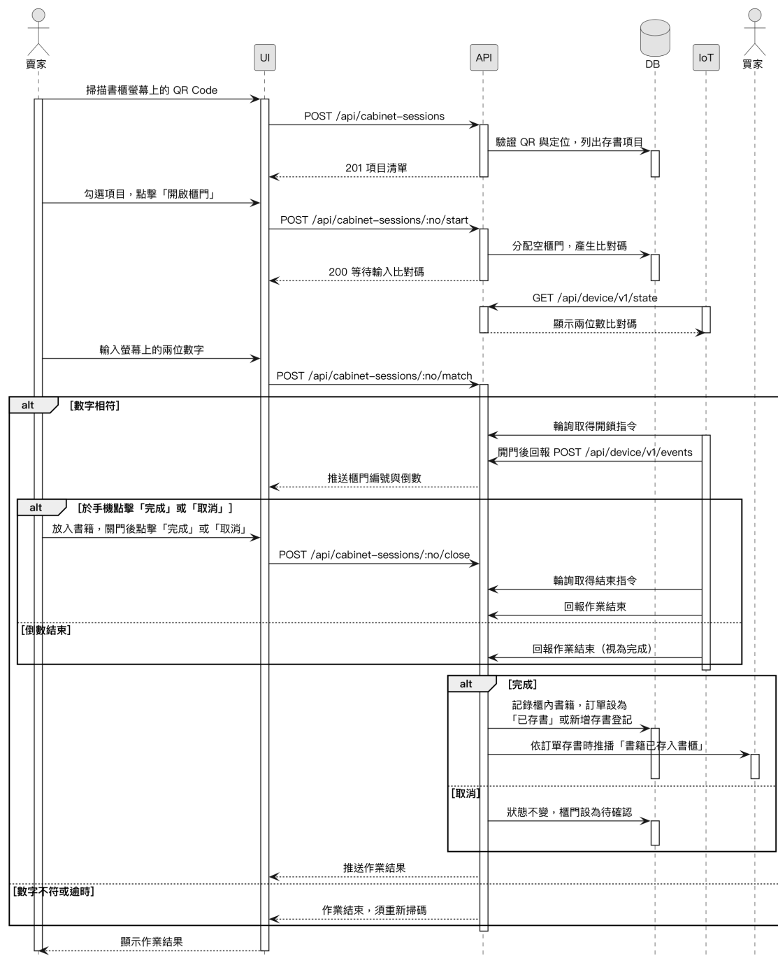
圖 6-1-5 賣家實體書櫃存書之循序圖
