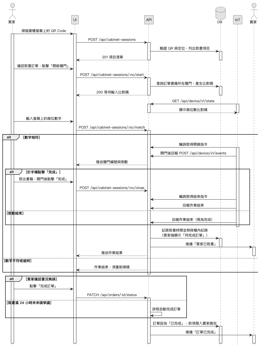
圖 6-1-7 買家實體書櫃取書與完成訂單之循序圖
