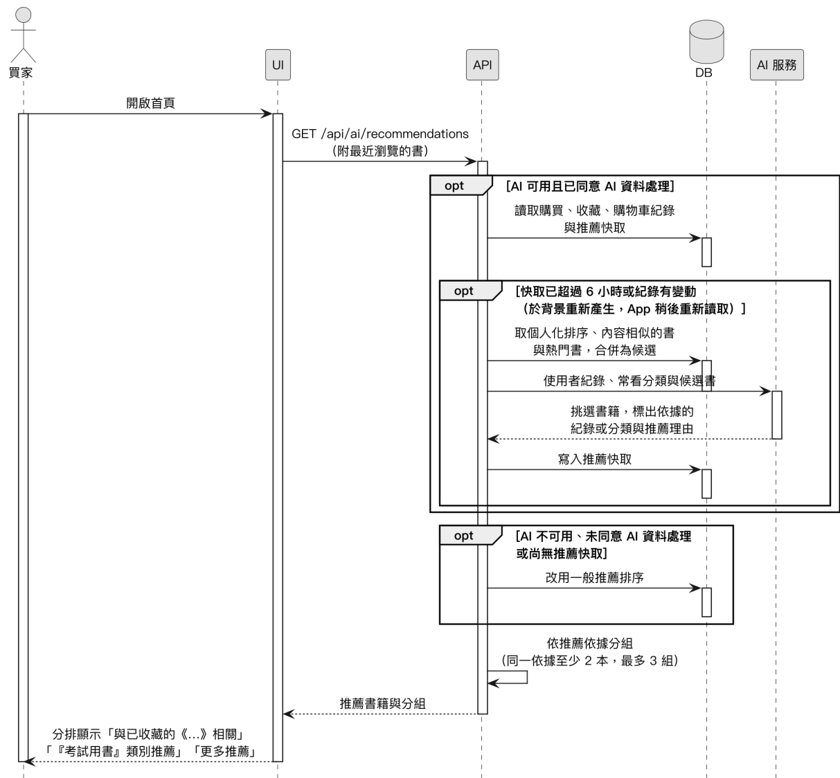
圖 6-1-23 個人化推薦之循序圖
