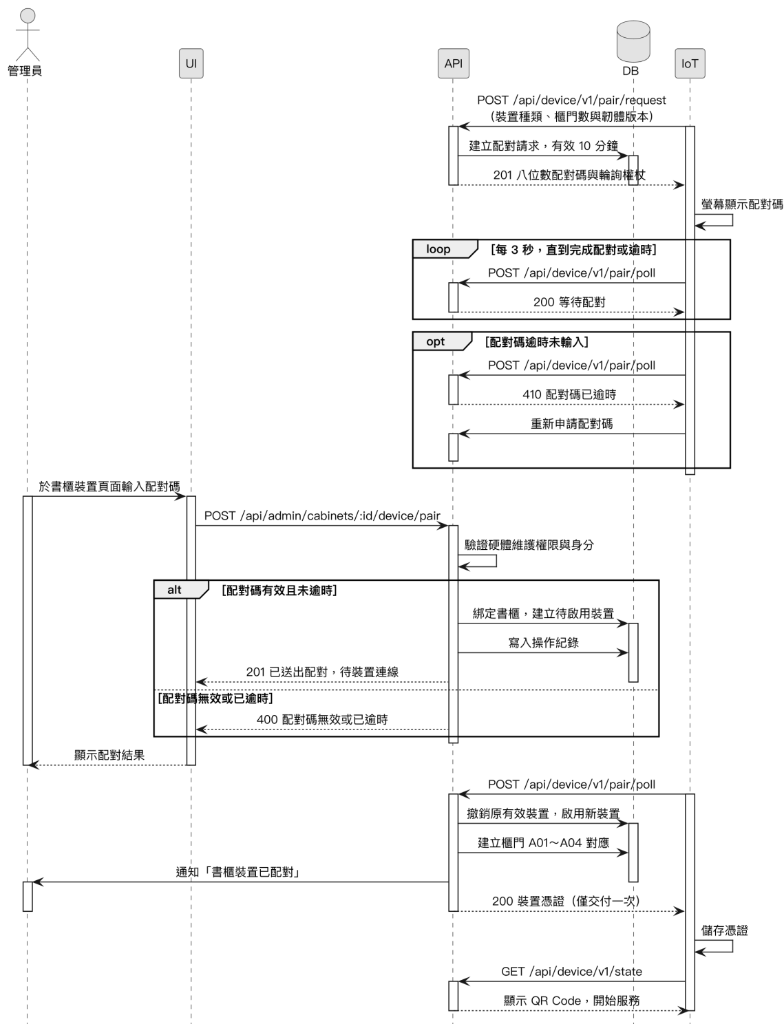
圖 6-1-30 書櫃裝置配對之循序圖
