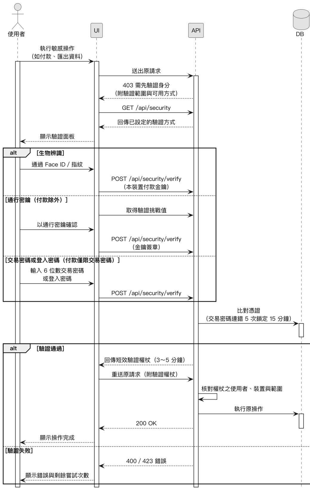
圖 6-1-15 敏感操作身分驗證之循序圖
