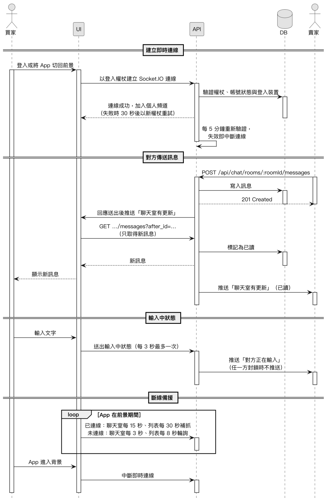
圖 6-1-28 聊天即時推送之循序圖
