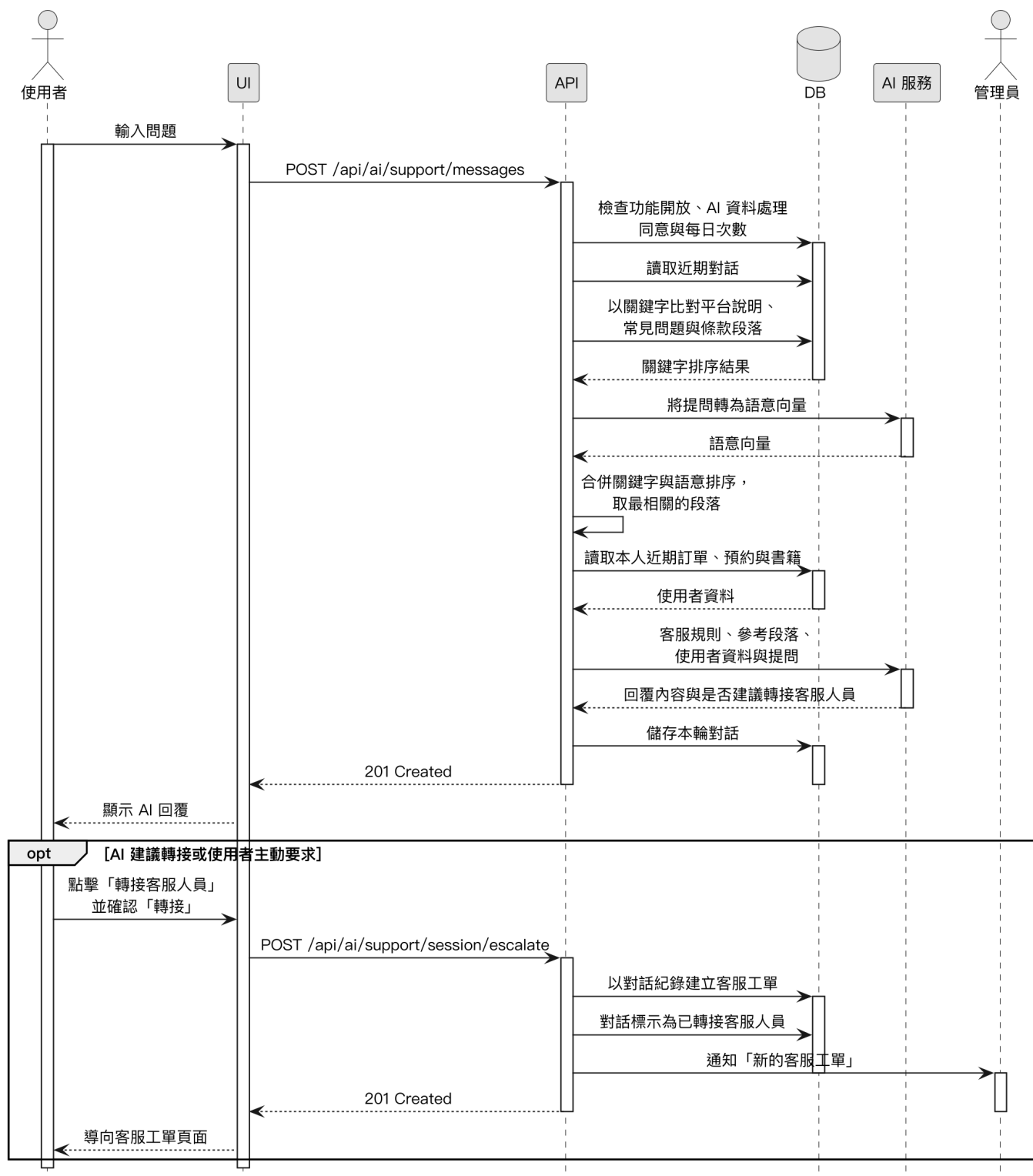
圖 6-1-11 AI 客服對話與轉接客服人員之循序圖
