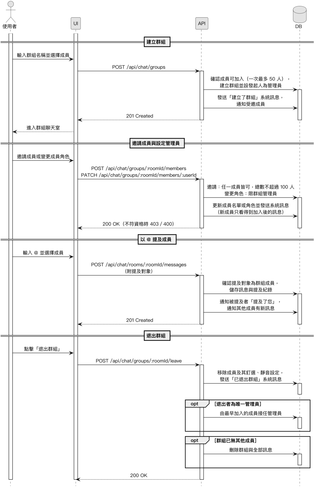
圖 6-1-19 群組聊天建立、管理與@提及之循序圖
