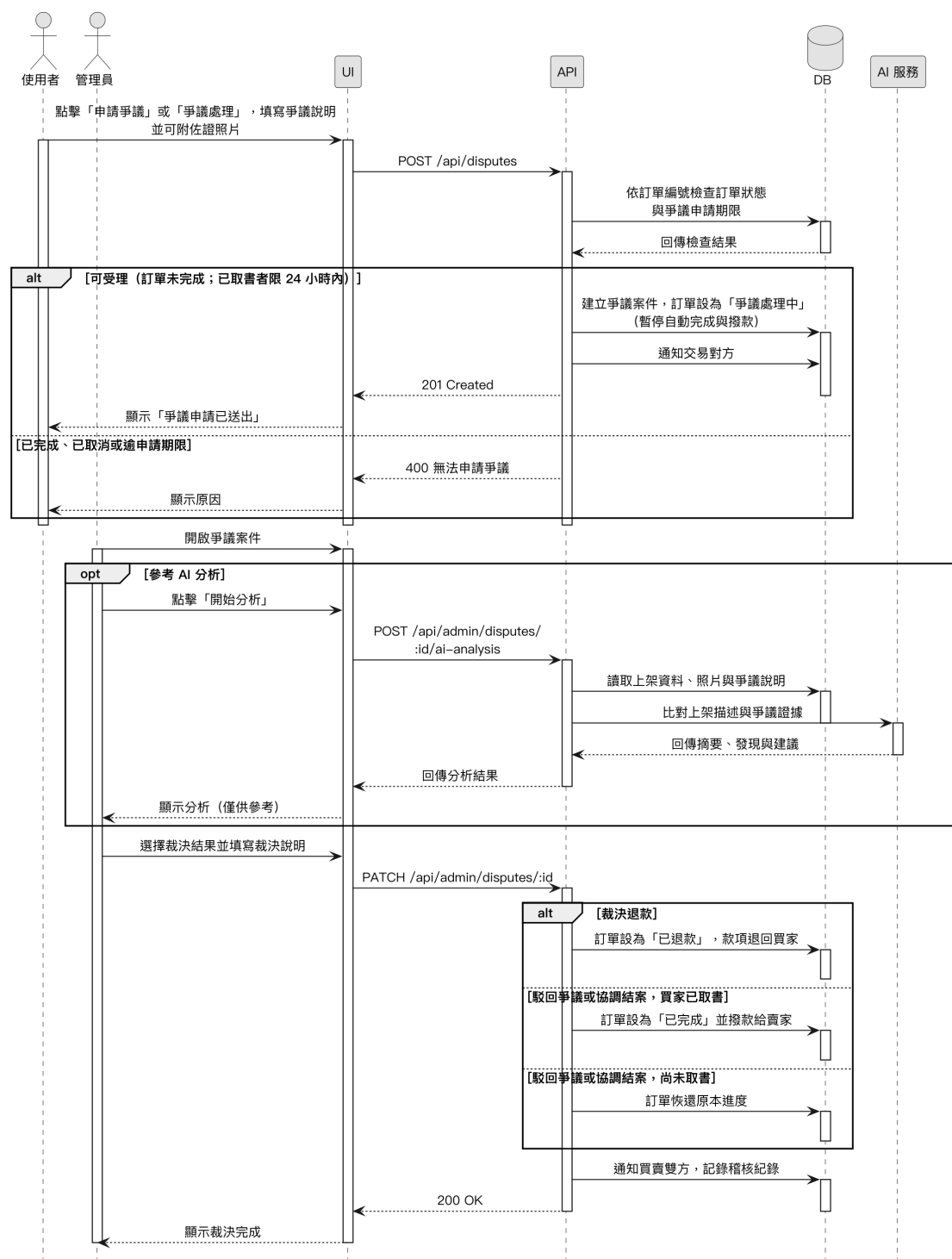
圖 6-1-8 訂單爭議與管理員裁決之循序圖
