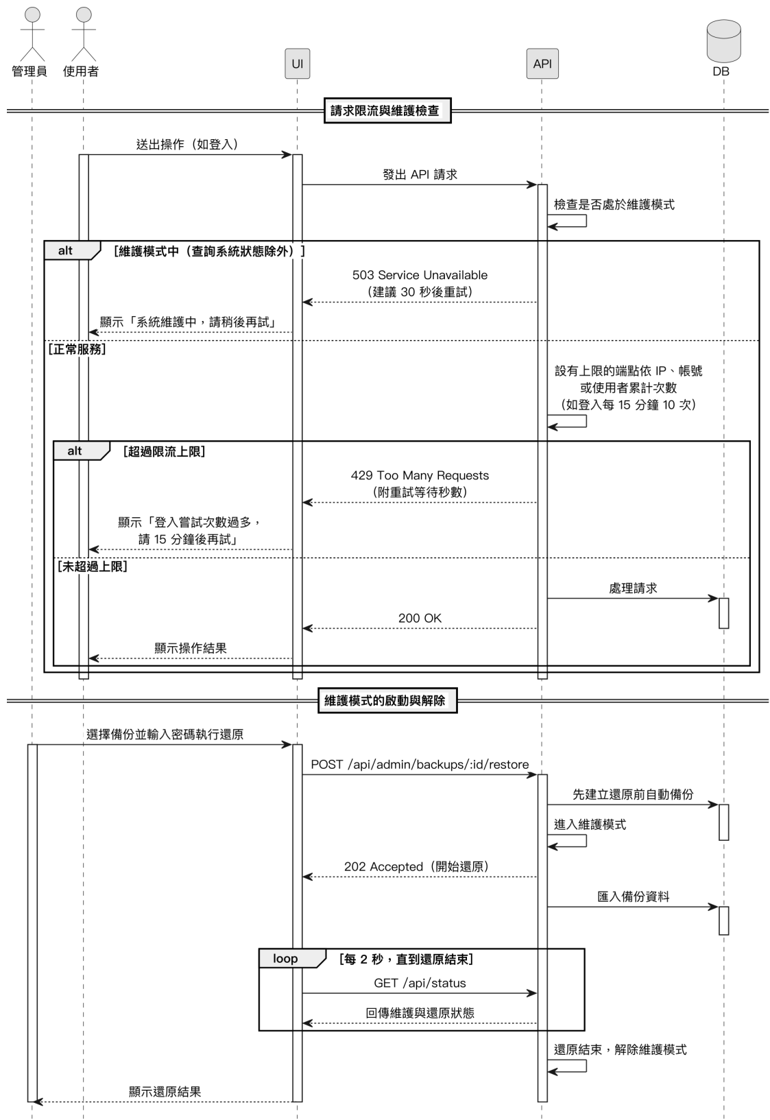
圖 6-1-25 系統限流與維護模式之循序圖
