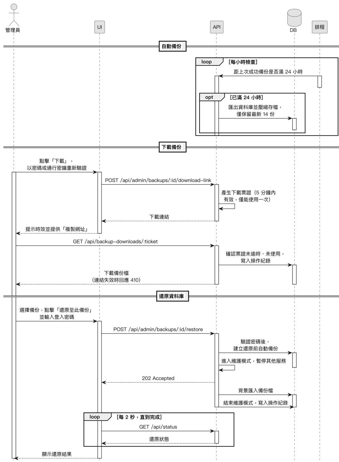
圖 6-1-22 資料庫備份與還原之循序圖
