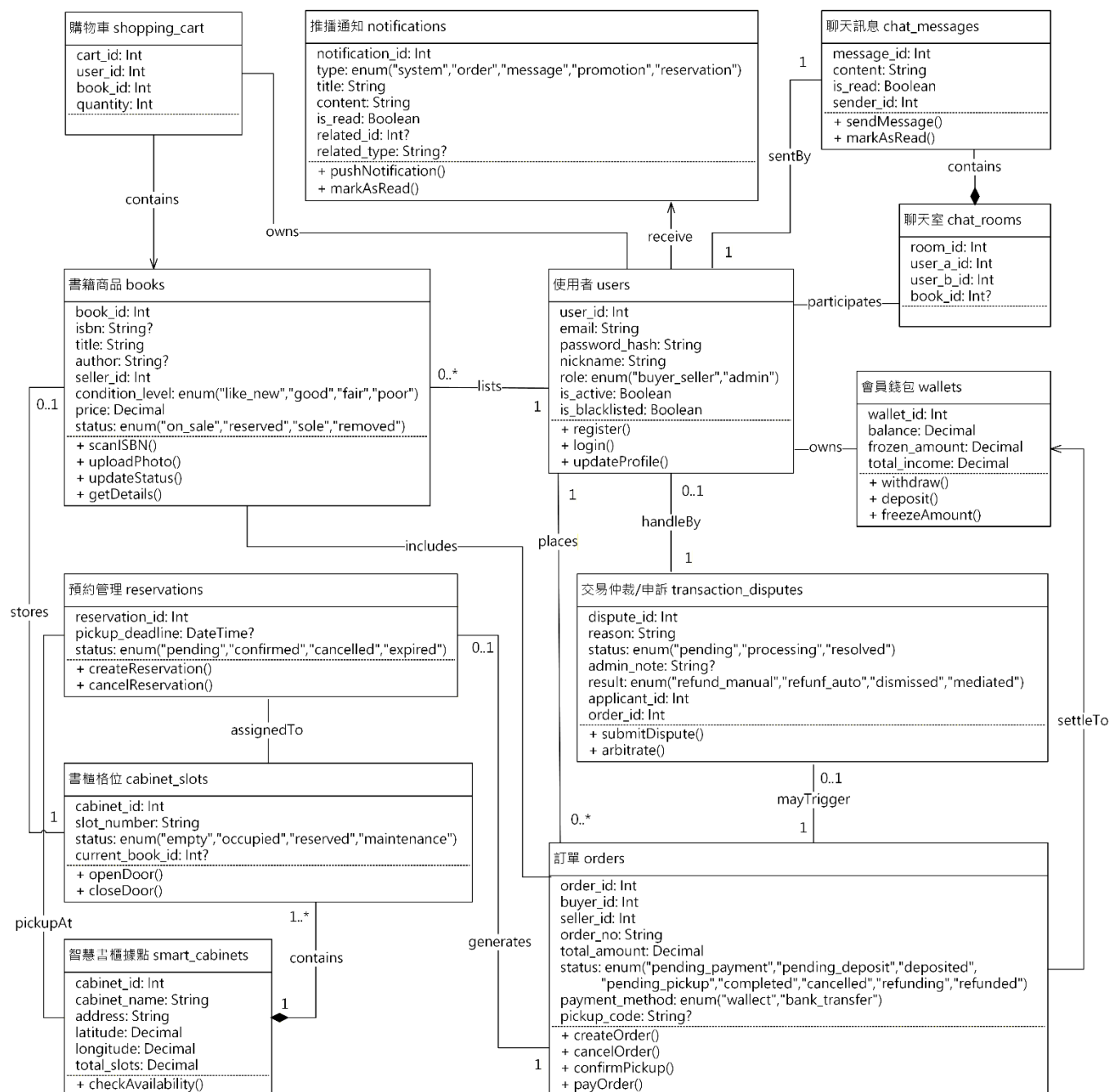
圖 6-2-1 設計類別圖
