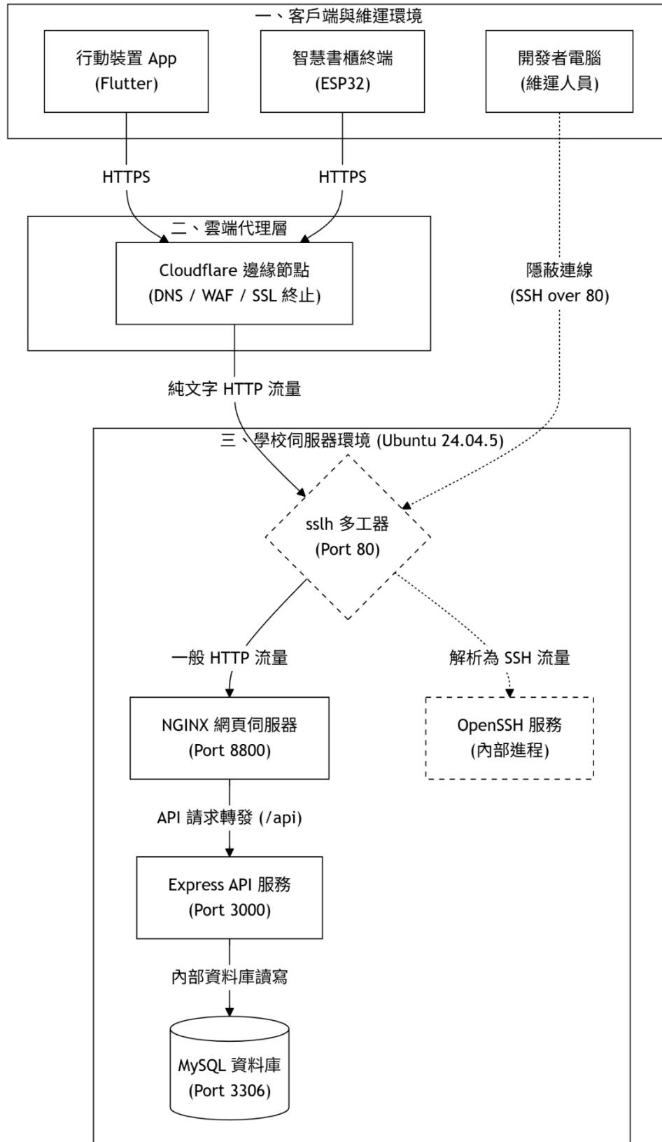
圖 7-1-1 佈署圖
