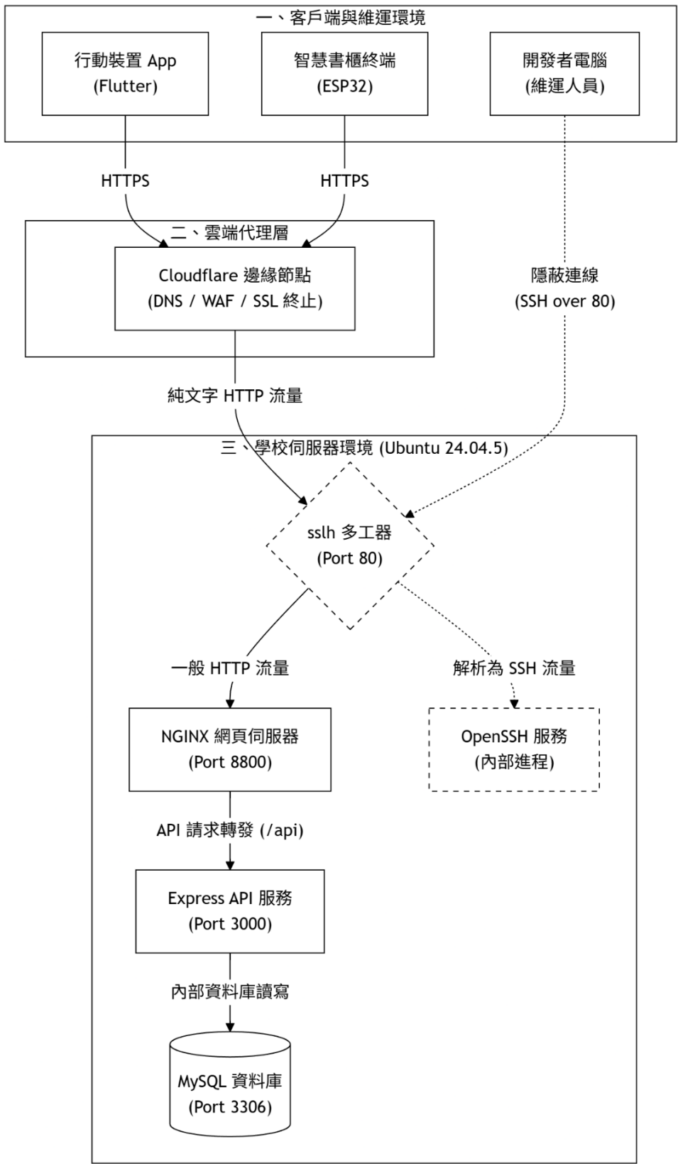
圖 7-1-1 佈署圖
