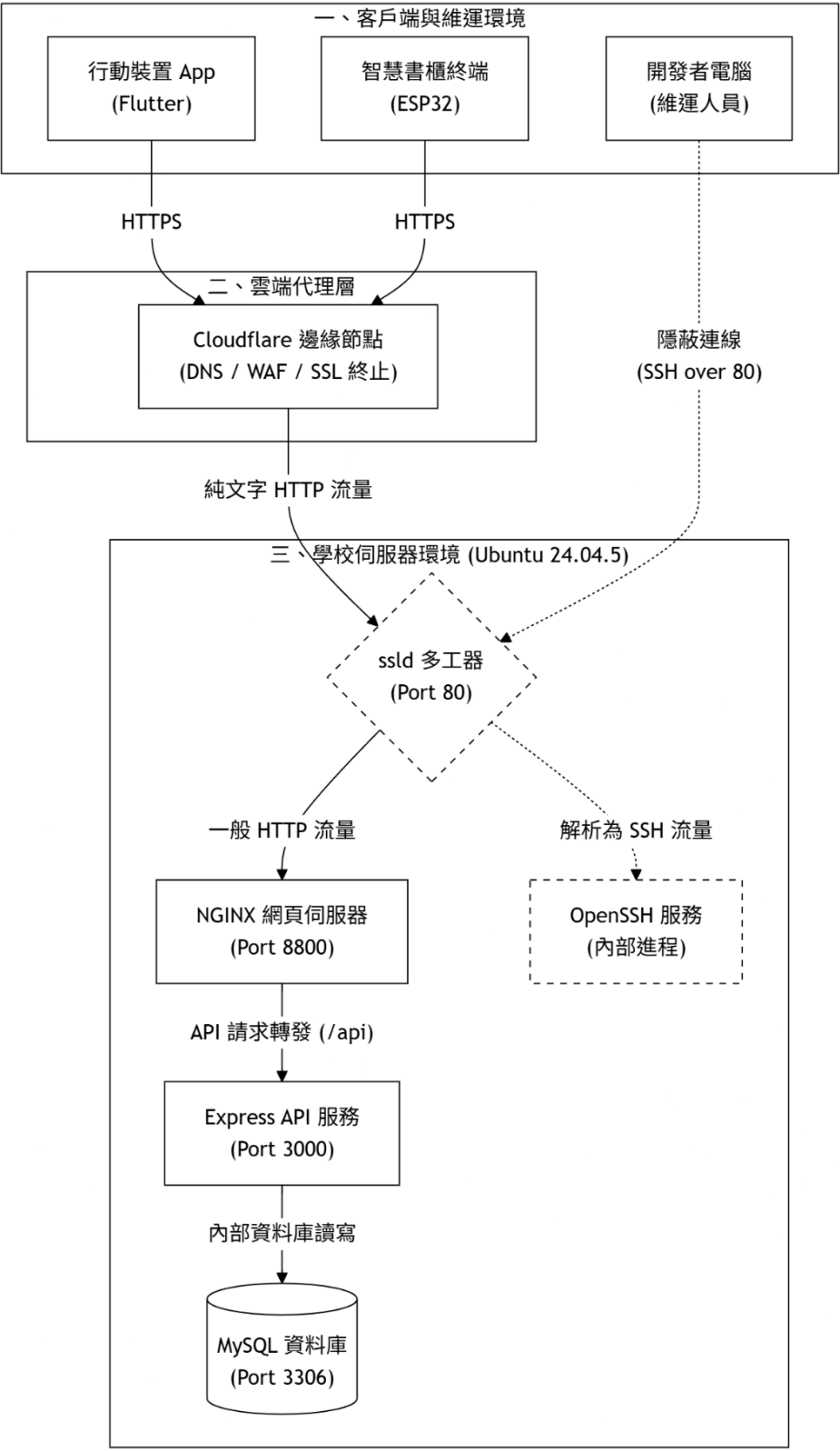
圖 7-1-1 佈署圖
