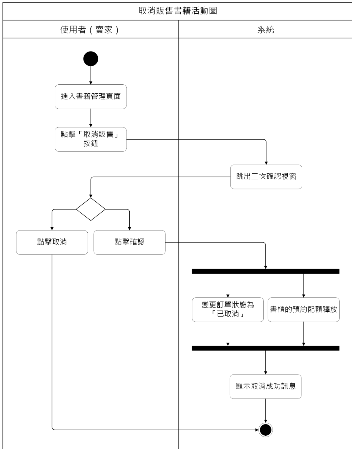
圖 5-3-3 取消販售書籍之活動圖
