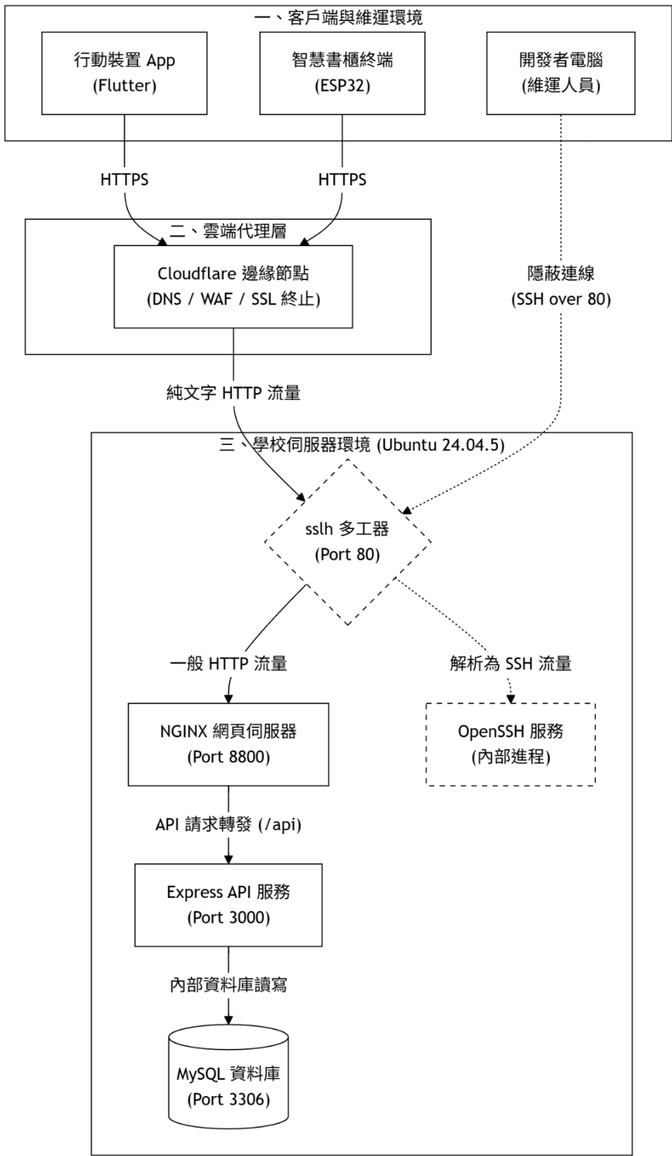
圖 7-1-1 佈署圖
