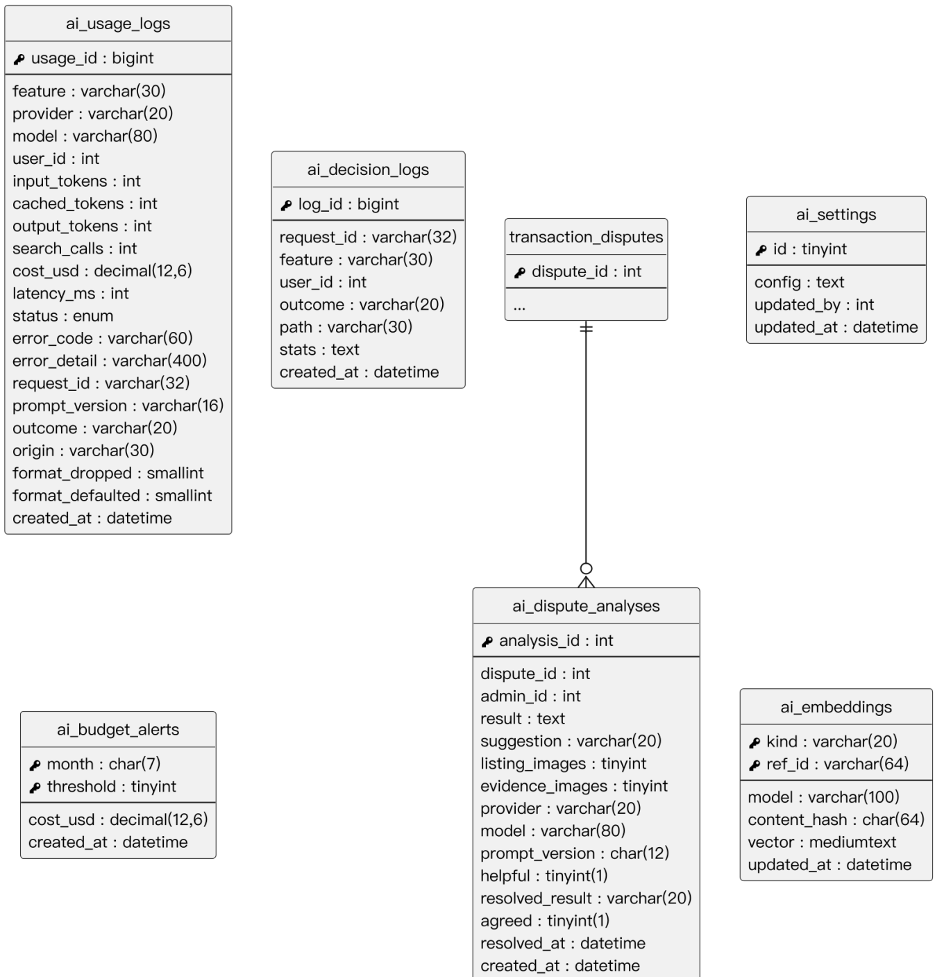
圖 8-1-15 AI 用量、設定與爭議分析模組 ER 圖
