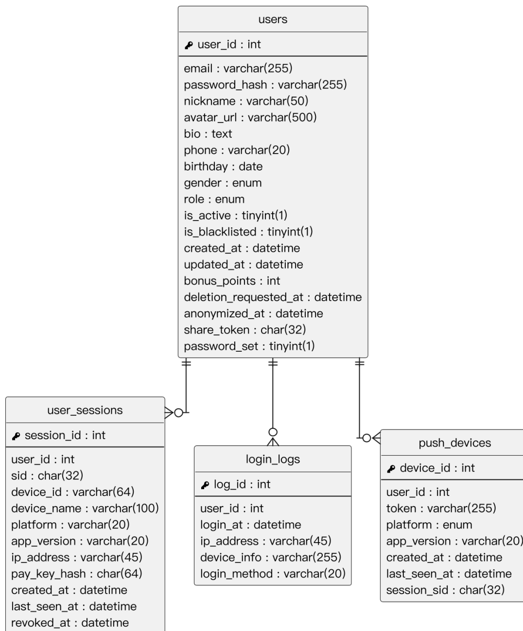
圖 8-1-1 使用者帳號與登入模組 ER 圖
