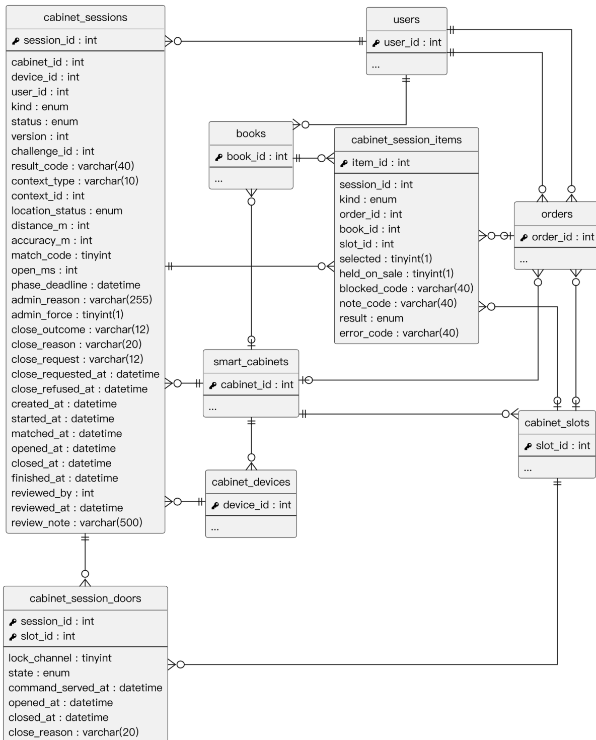
圖 8-1-9 書櫃作業模組 ER 圖
