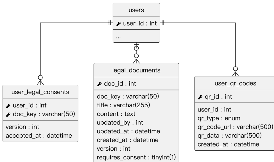
圖 8-1-4 條款同意與 QR Code 模組 ER 圖
