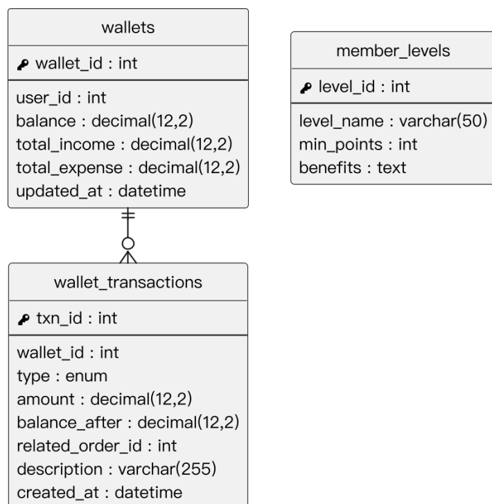
圖 8-1-12 錢包與會員成長模組 ER 圖
