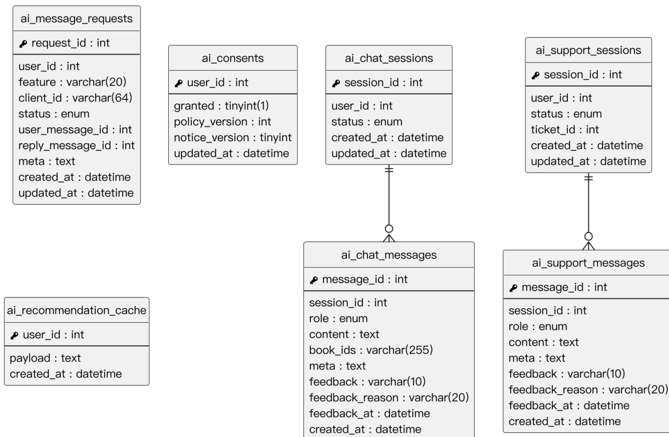
圖 8-1-13 AI 對話、同意與推薦快取模組 ER 圖
