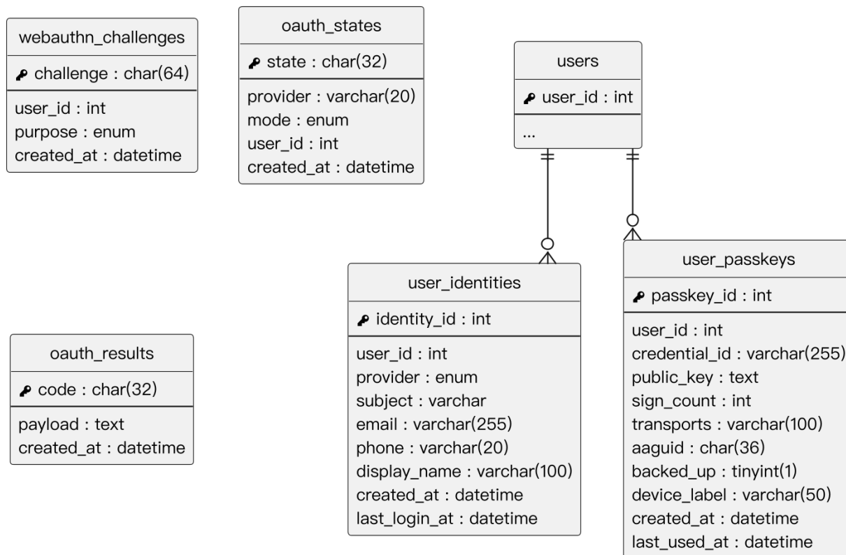
圖 8-1-2 通行密鑰與第三方登入模組 ER 圖
