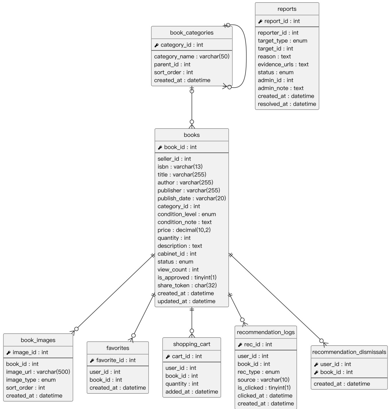
圖 8-1-5 書籍與商品模組 ER 圖
