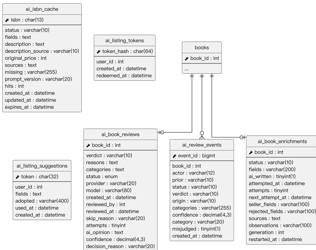
圖 8-1-14 AI 上架輔助、審核與書目補齊模組 ER 圖
