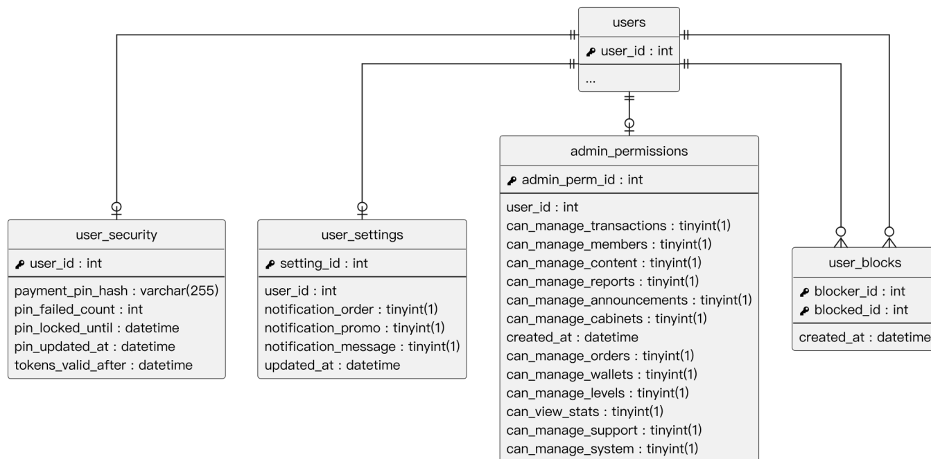
圖 8-1-3 帳號安全與偏好設定模組 ER 圖
