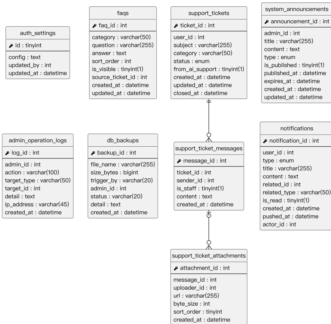
圖 8-1-16 客服、公告與後台模組 ER 圖
