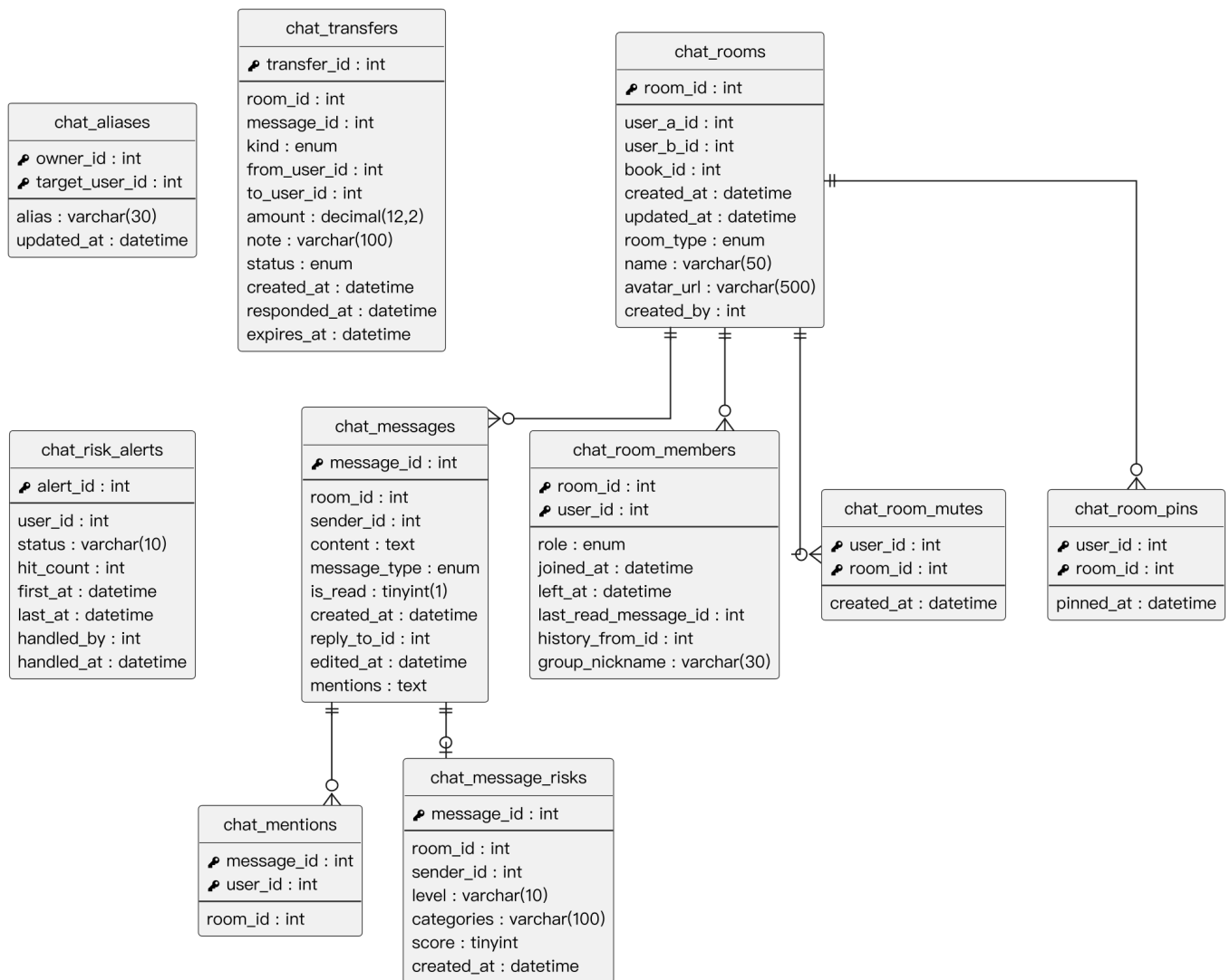
圖 8-1-11 聊天與社交模組 ER 圖
