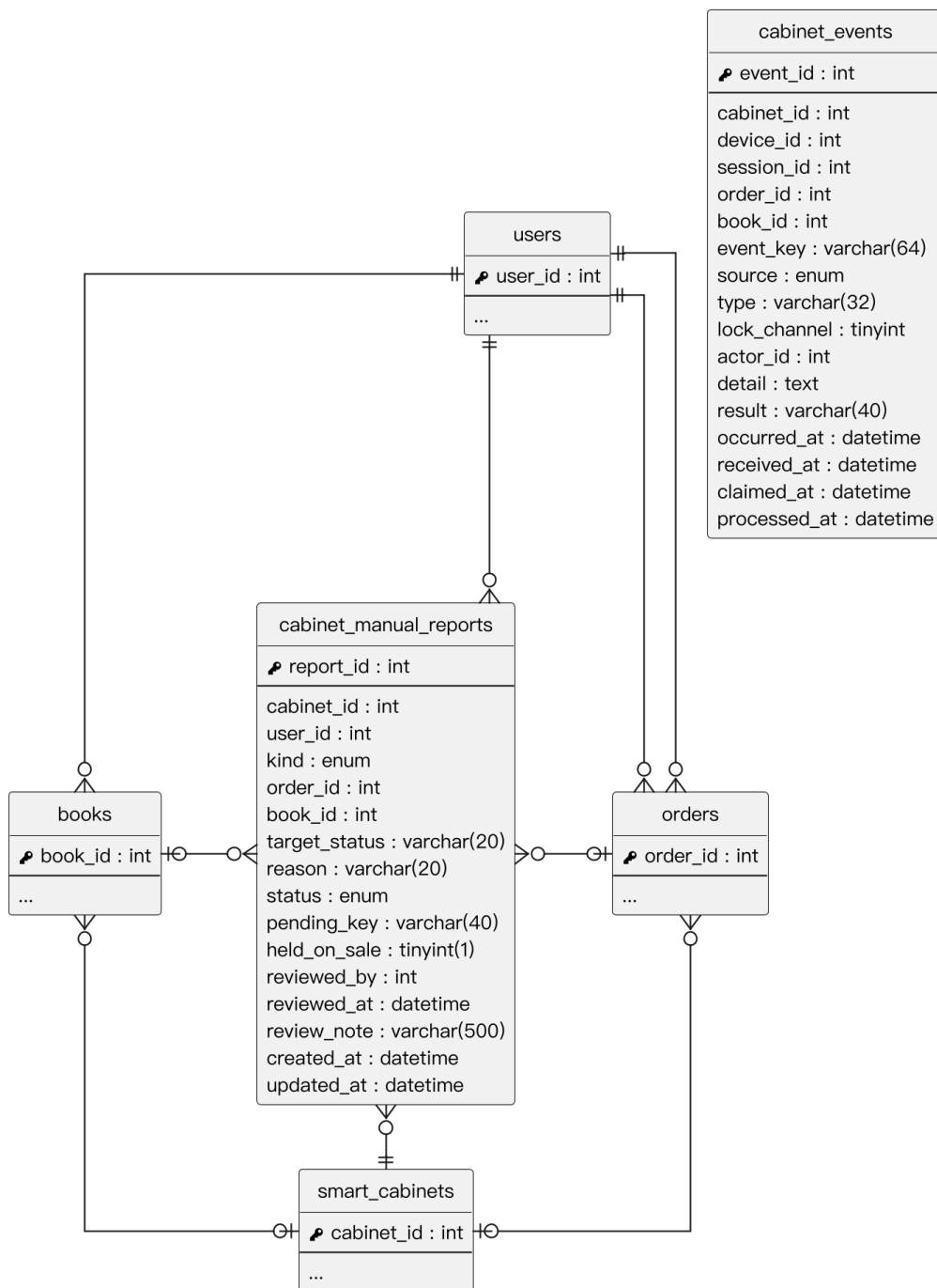
圖 8-1-10 書櫃手動回報與事件紀錄模組 ER 圖
