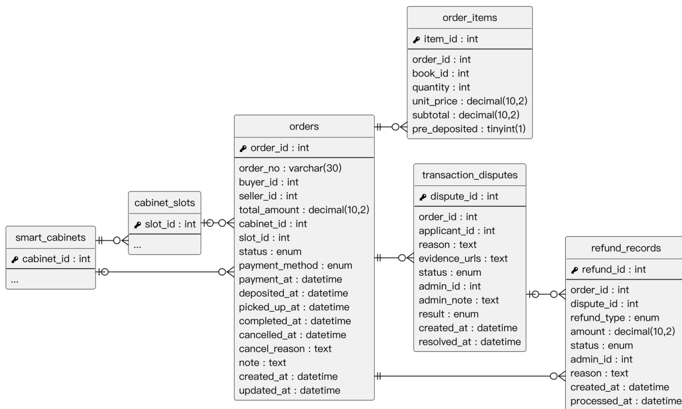
圖 8-1-6 交易訂單與退款模組 ER 圖
