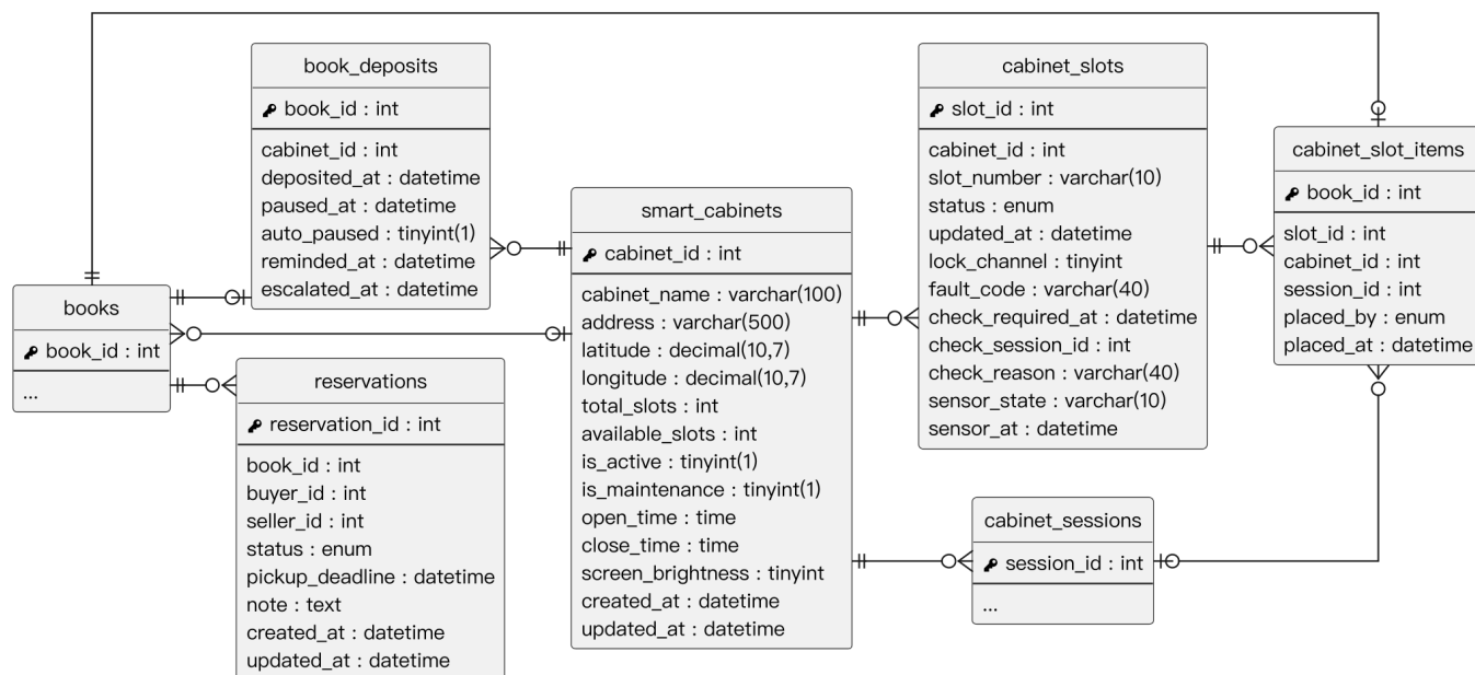
圖 8-1-7 智慧書櫃、存書與預約模組 ER 圖
