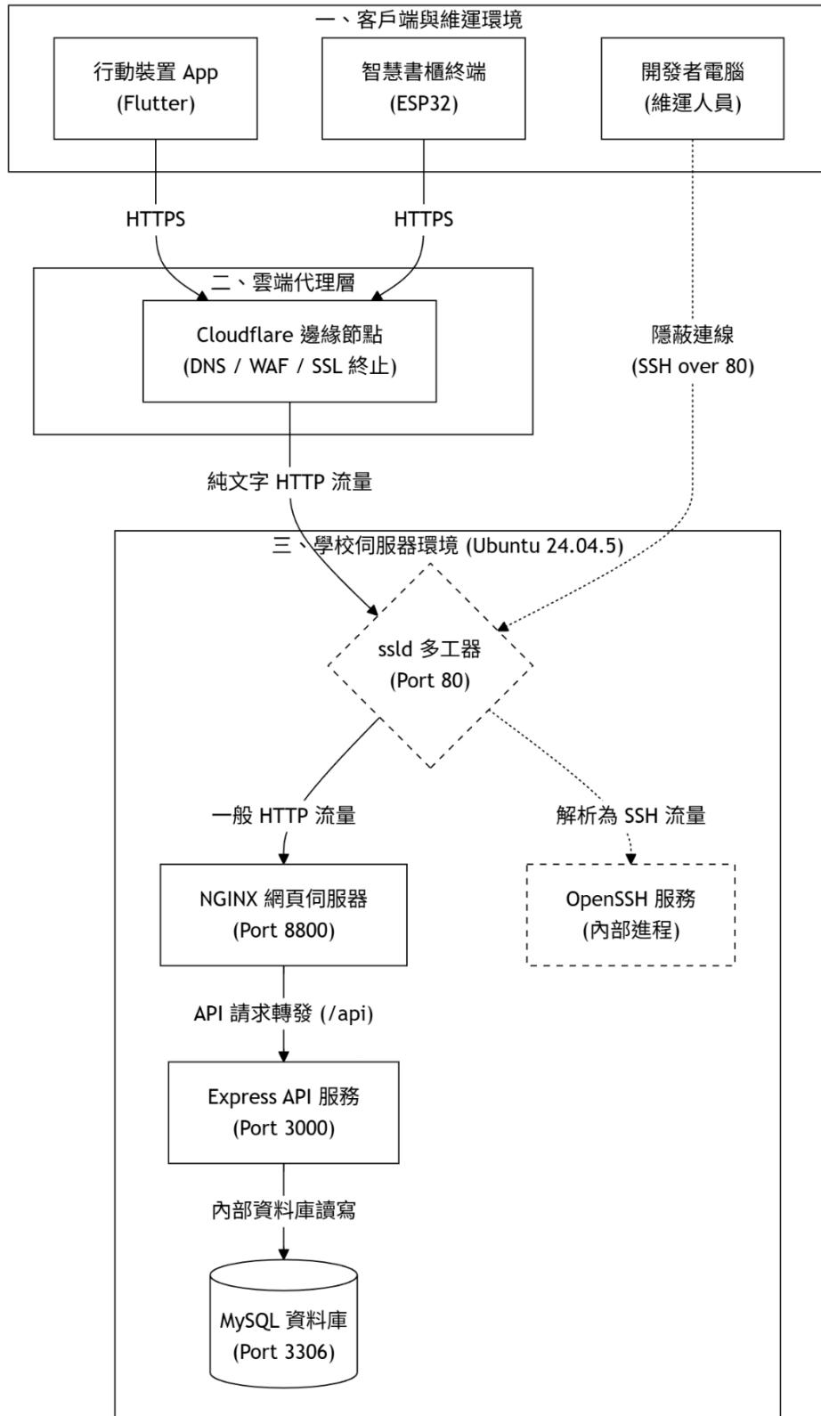
圖 7-1-1 佈署圖
