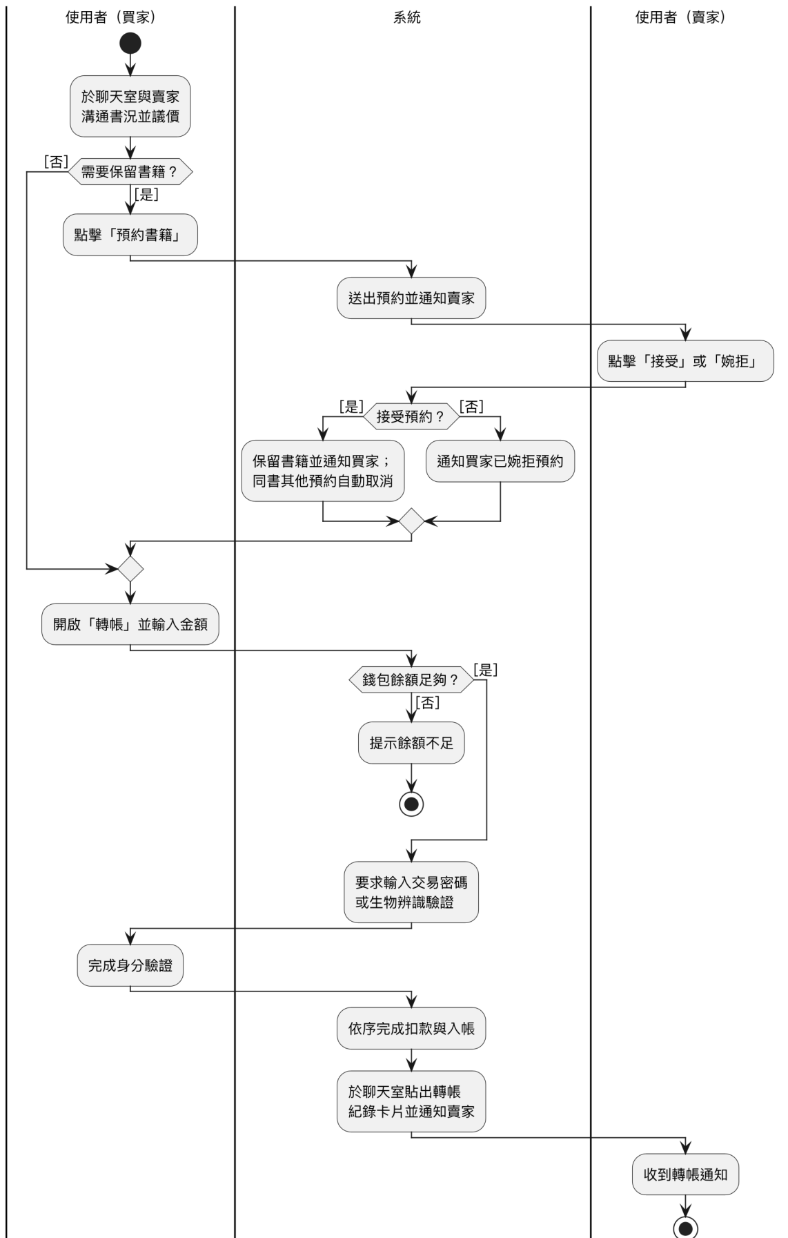
圖 5-3-9 聊天協商、預約與站內轉帳之活動圖
