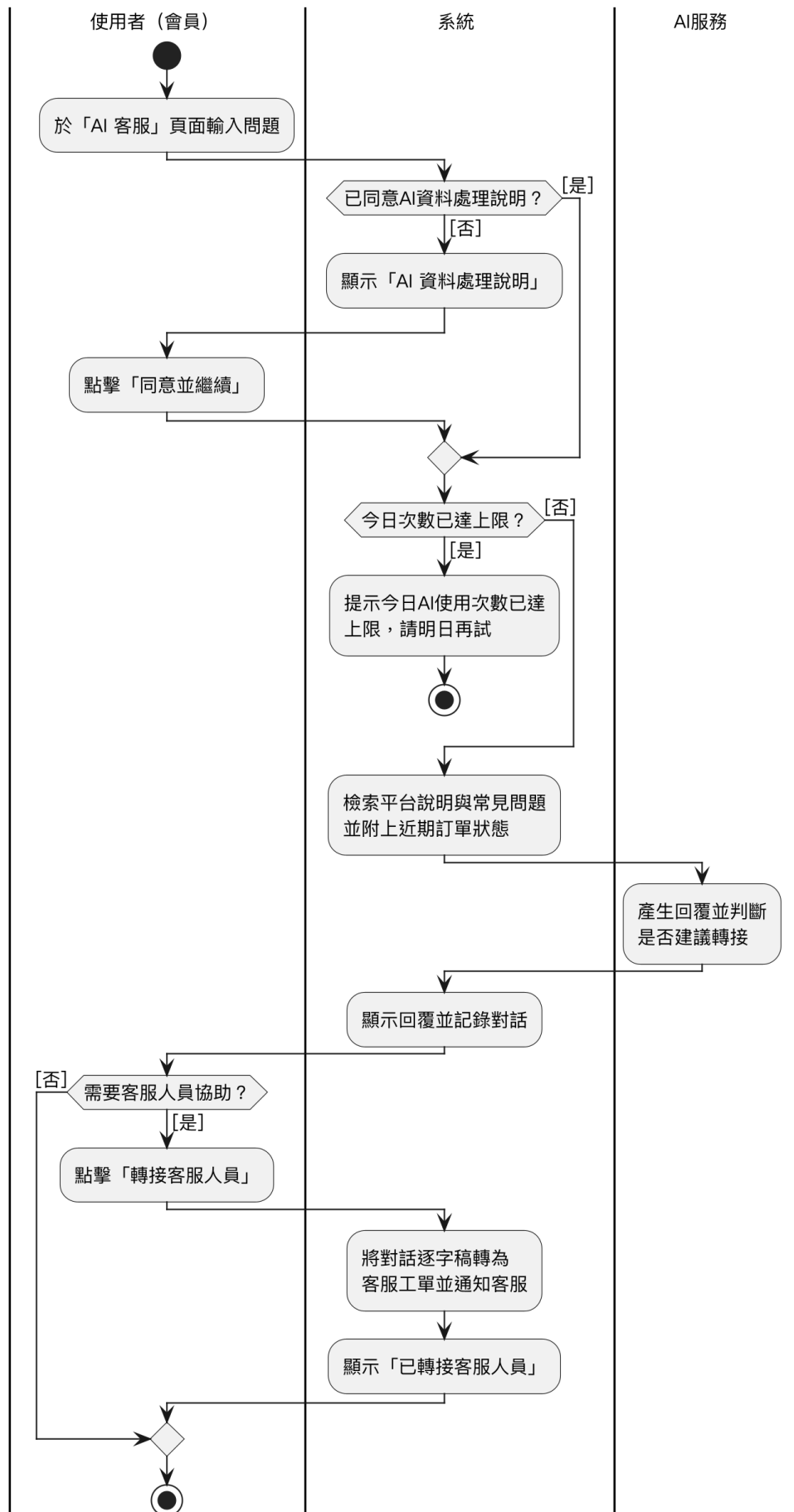
圖 5-3-10 AI 客服對話與轉接客服人員之活動圖
