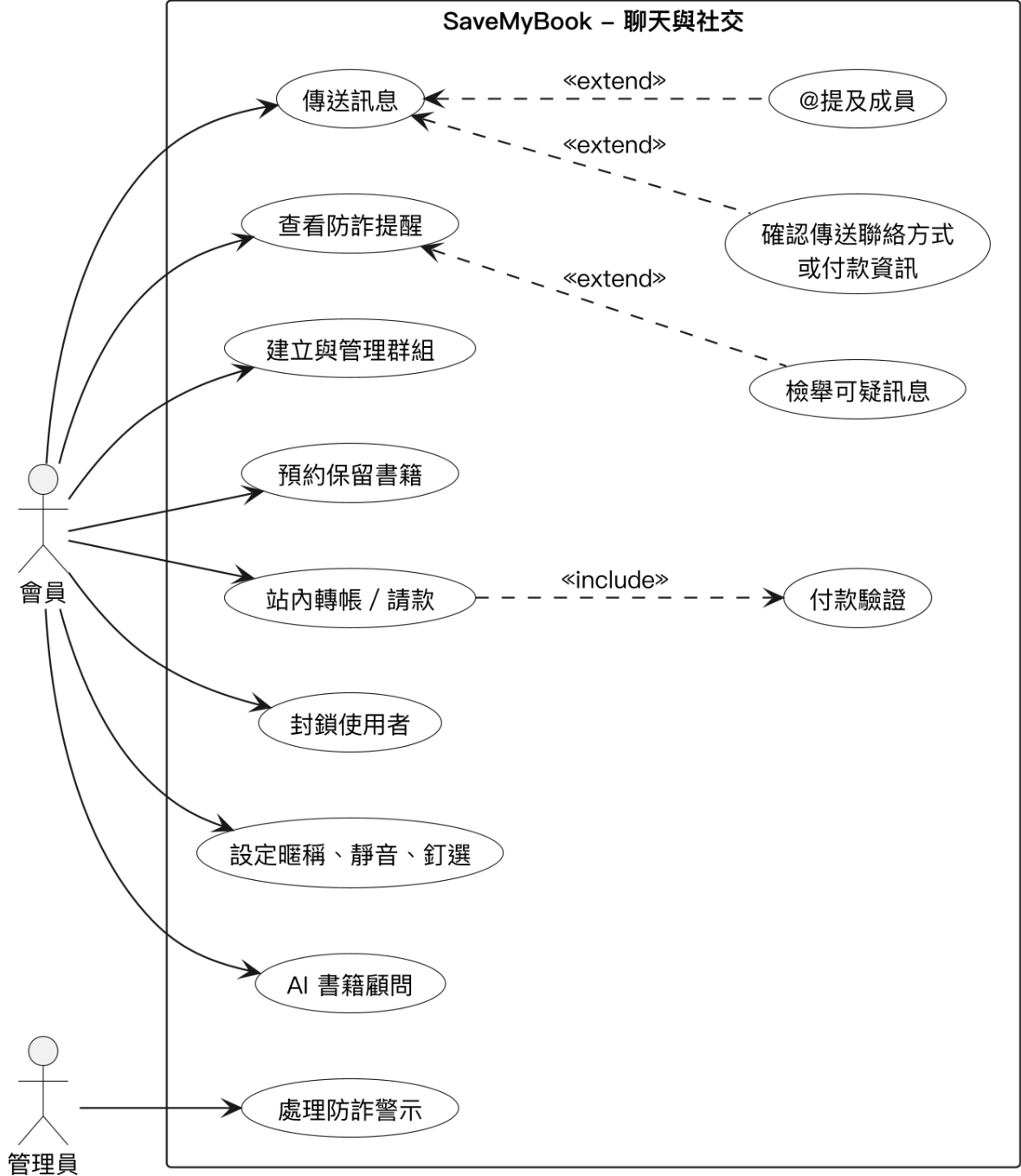
圖 5-2-4 聊天與社交模組之使用個案圖
