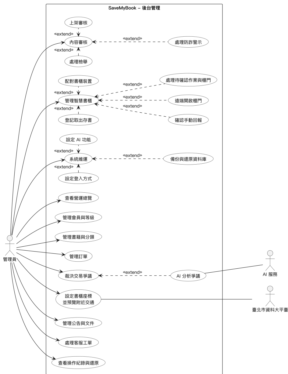
圖 5-2-6 後台管理模組之使用個案圖
