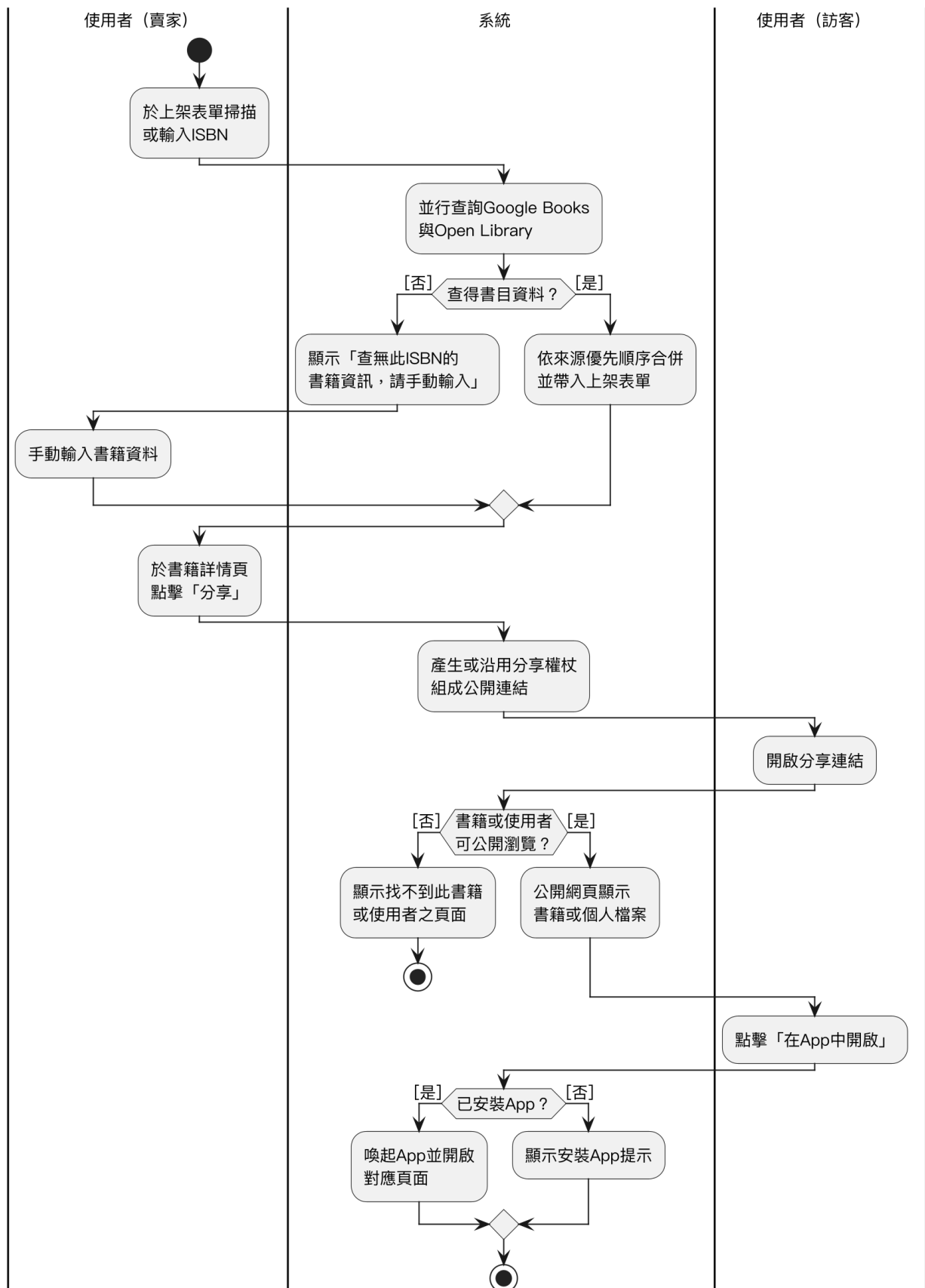
圖 5-3-24 ISBN 查詢與書籍/個人分享連結之活動圖
