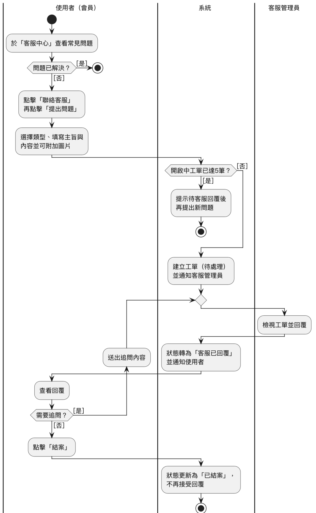
圖 5-3-12 客服工單之活動圖
