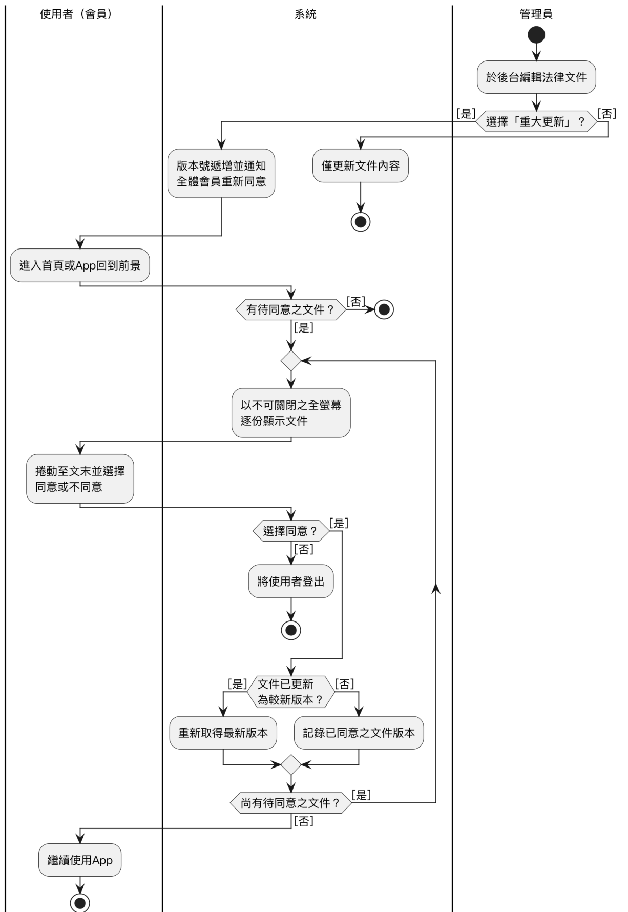
圖 5-3-18 法律文件同意（服務條款/隱私權政策）之活動圖
