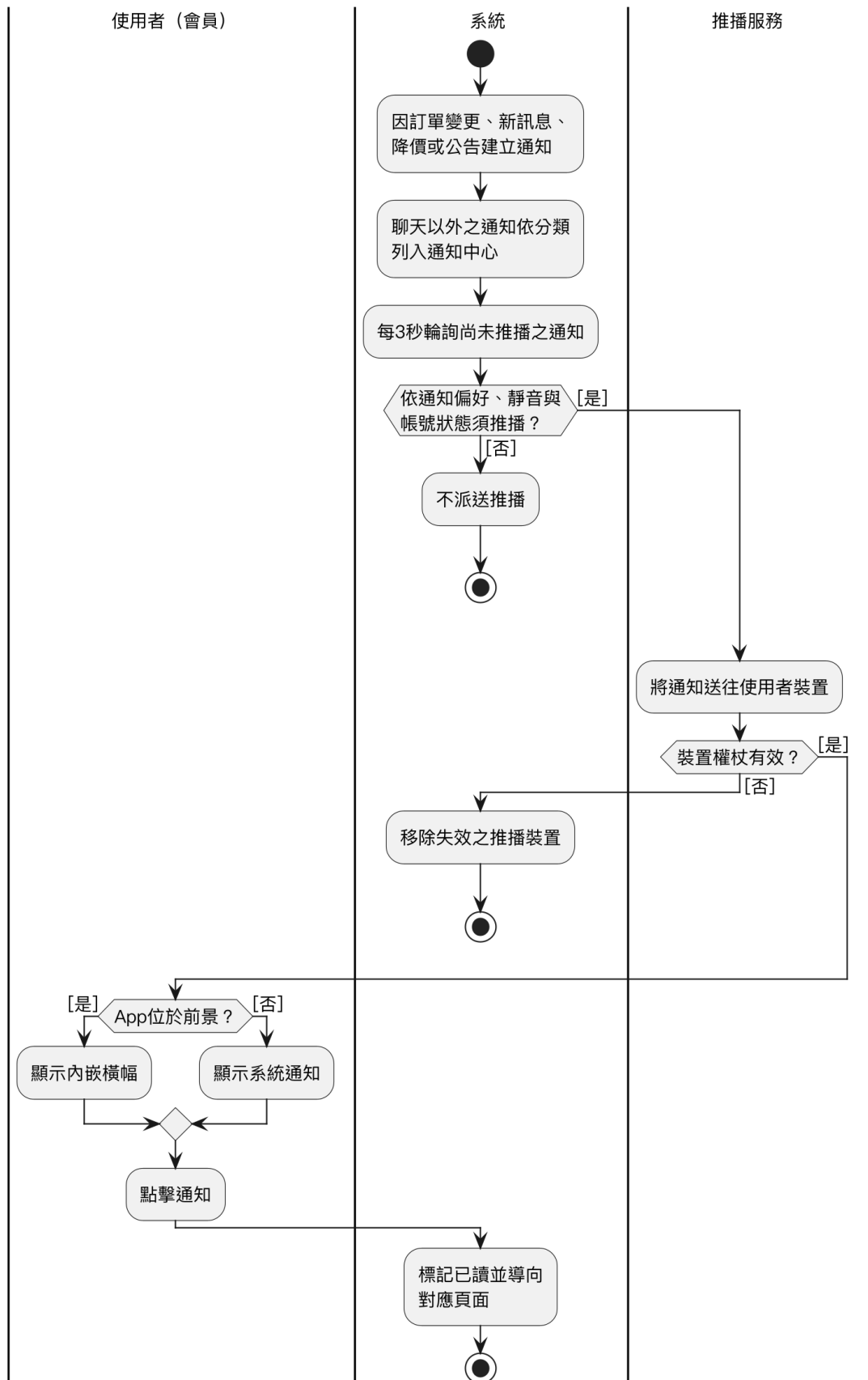
圖 5-3-20 站內通知與 App 推播之活動圖
