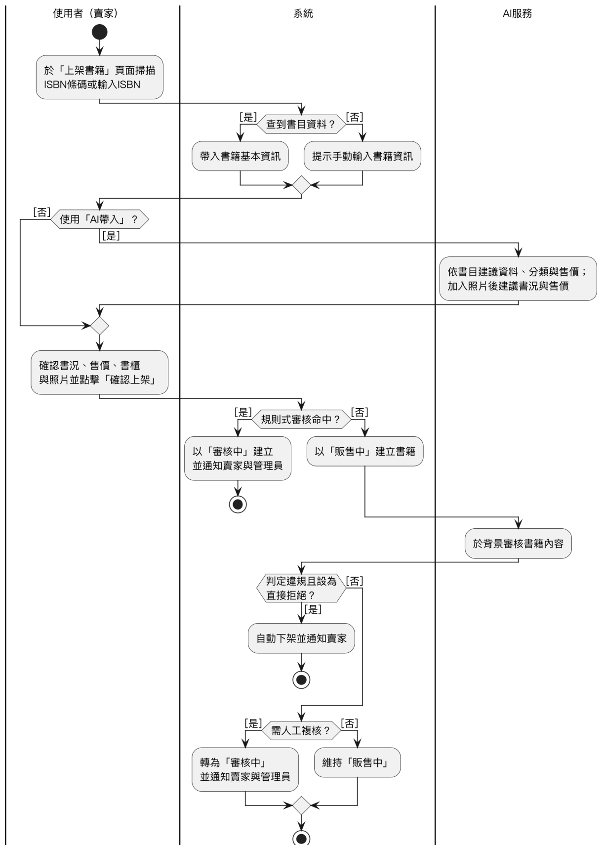
圖 5-3-1 上架書籍（含 AI 輔助）之活動圖
