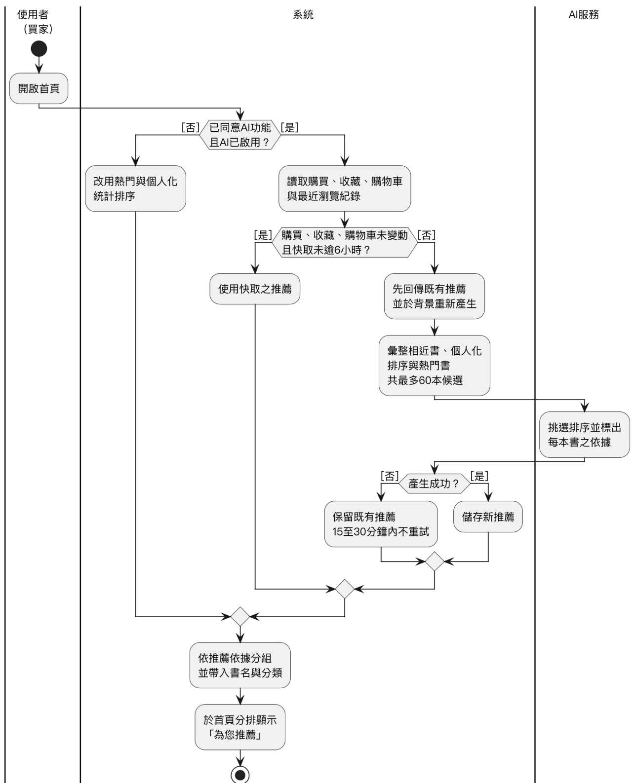
圖 5-3-23 個人化推薦（AI 與非 AI 後備）之活動圖
