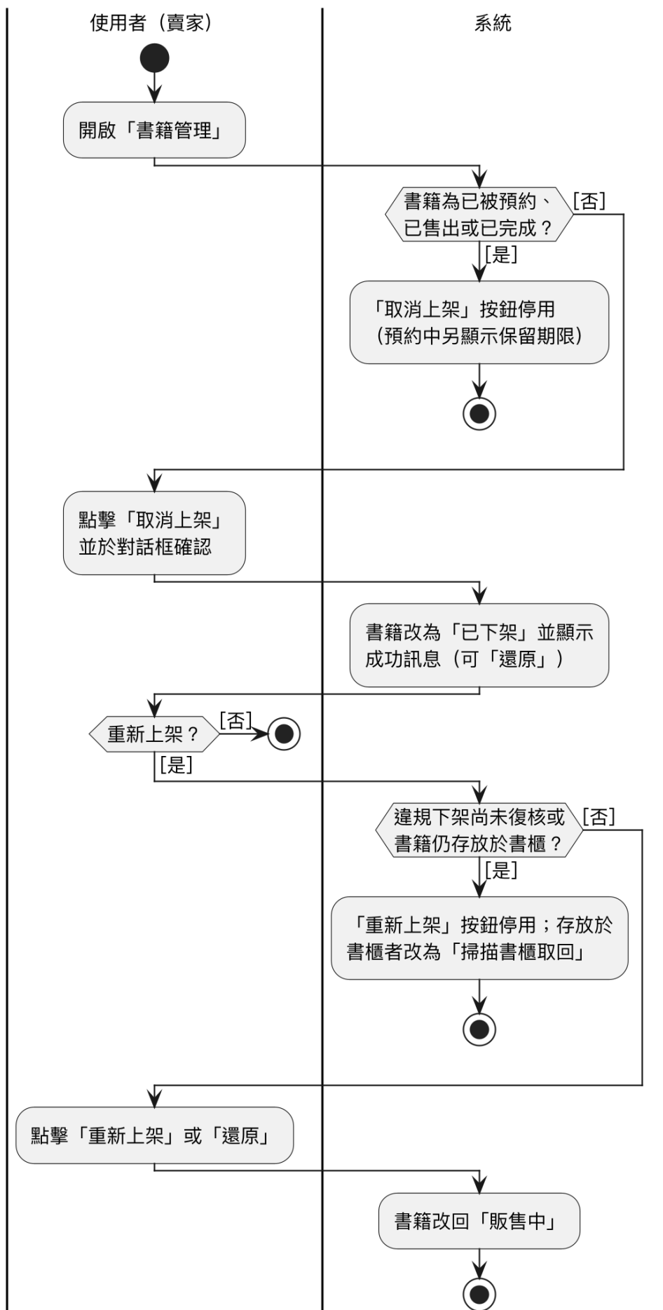
圖 5-3-3 取消(下架)/重新上架書籍之活動圖
