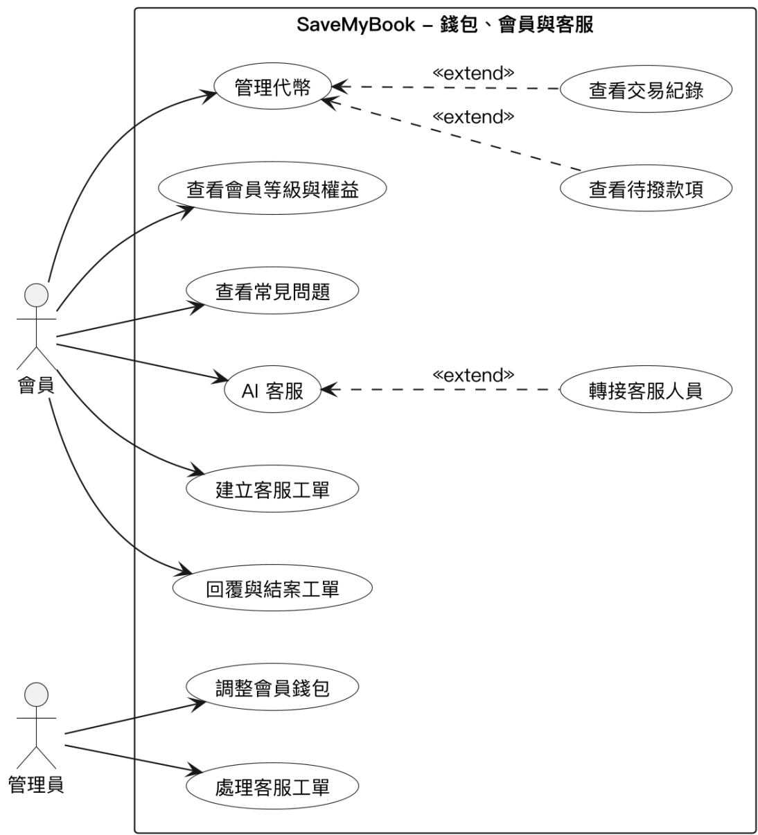
圖 5-2-5 錢包、會員成長與客服模組之使用個案圖
