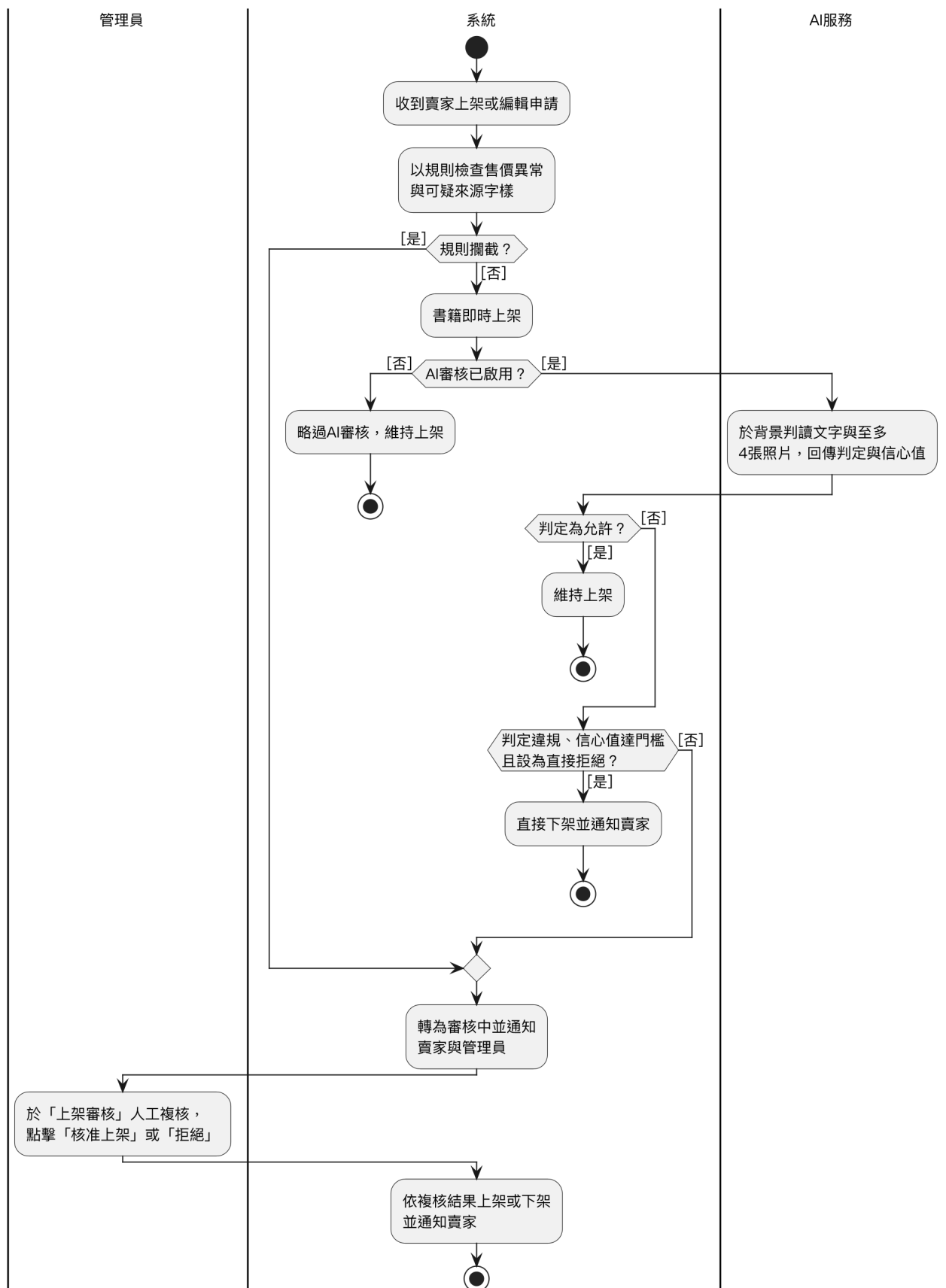
圖 5-3-13 AI 輔助上架內容審核（規則式+AI 雙層）之活動圖
