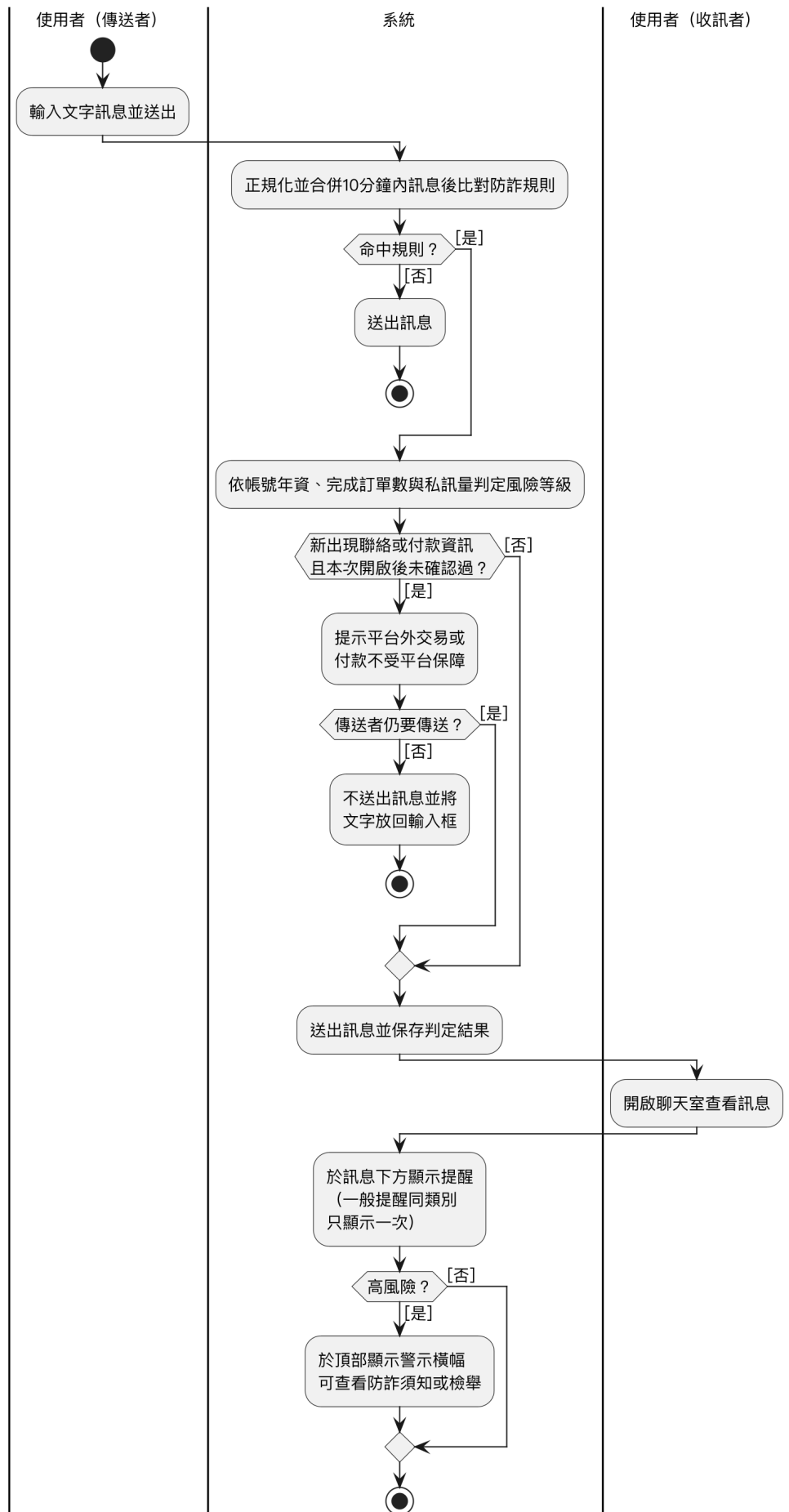
圖 5-3-27 聊天防詐提醒與傳送確認之活動圖
