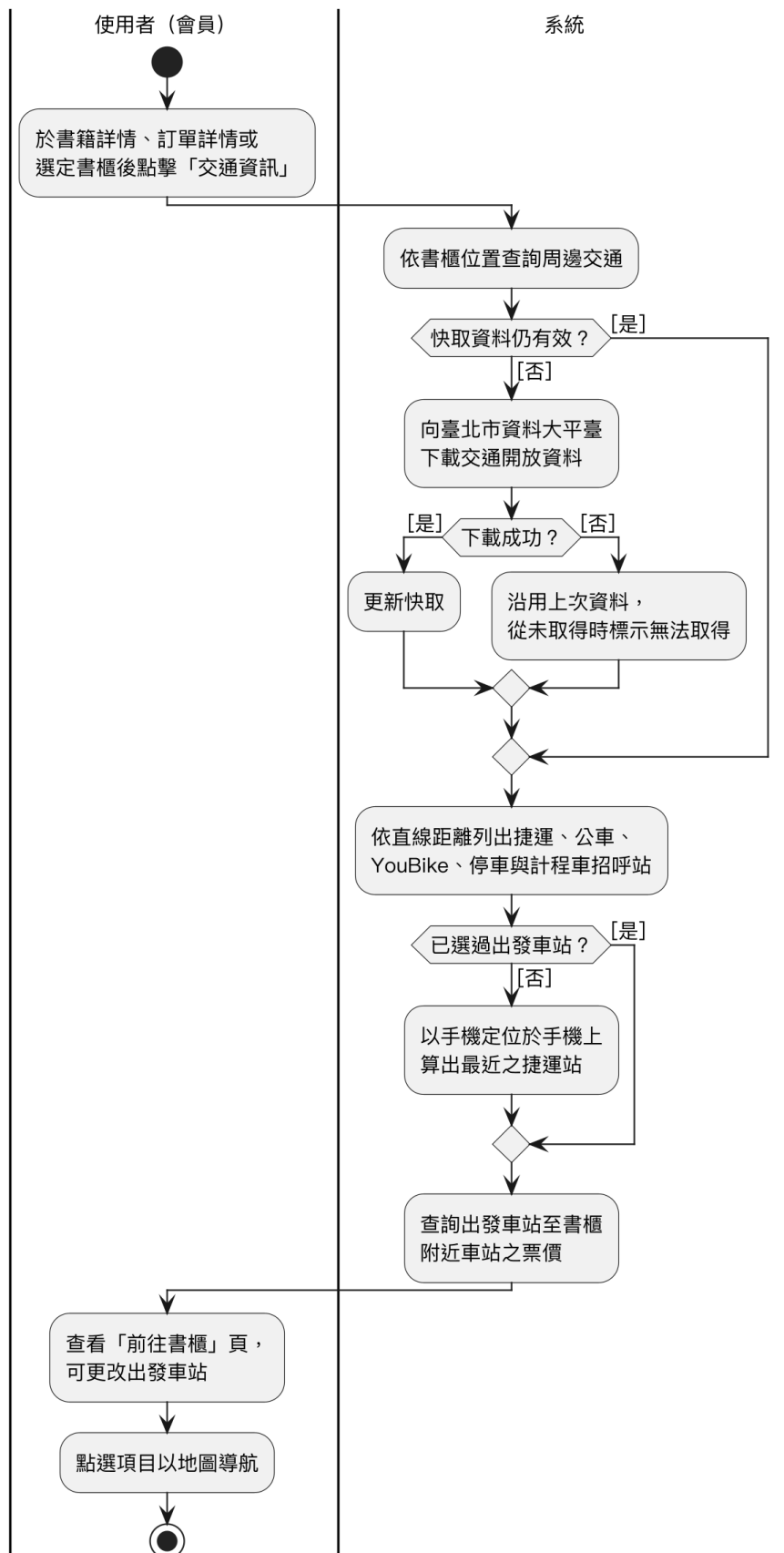
圖 5-3-35 查看前往書櫃交通資訊之活動圖
