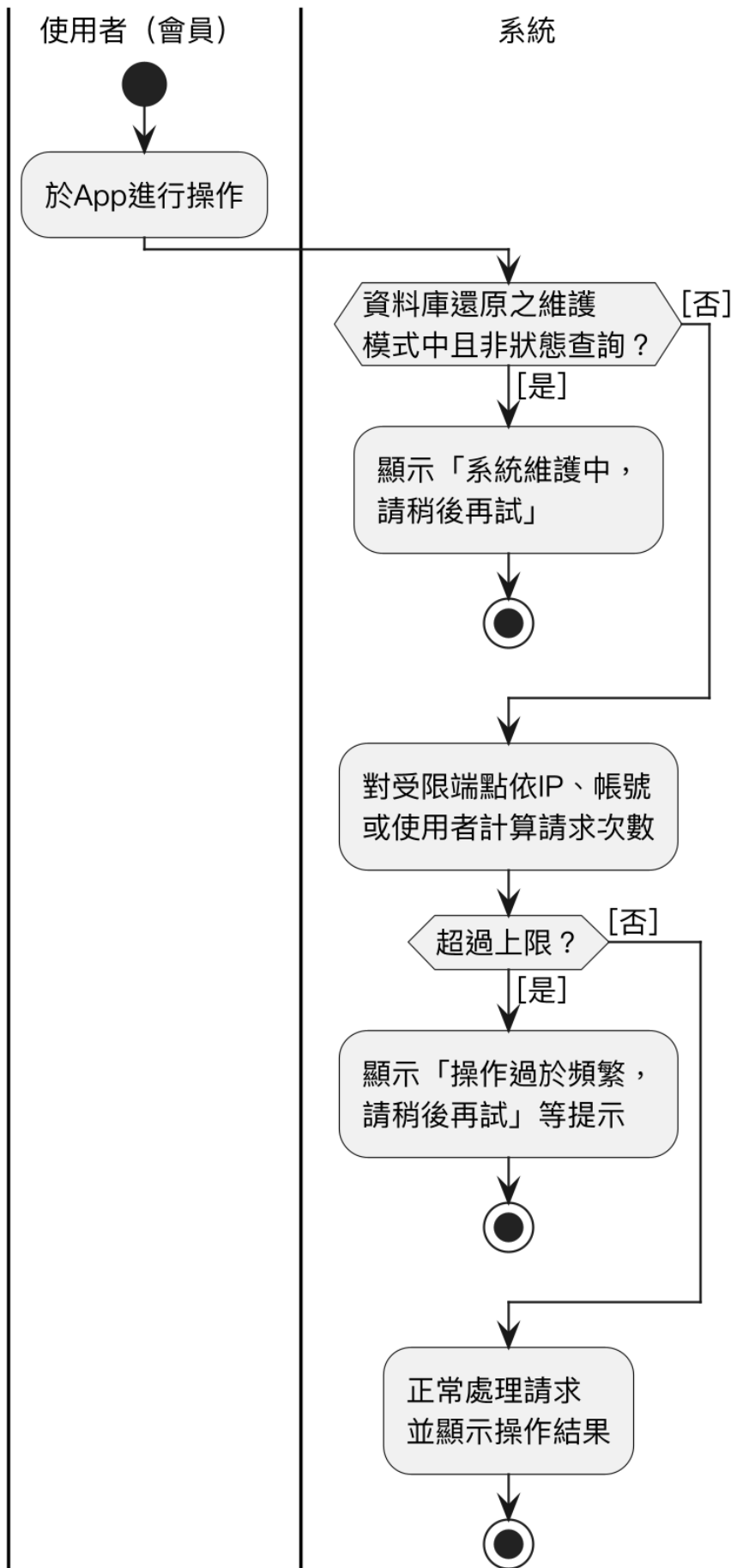
圖 5-3-25 系統限流與維護模式之活動圖
