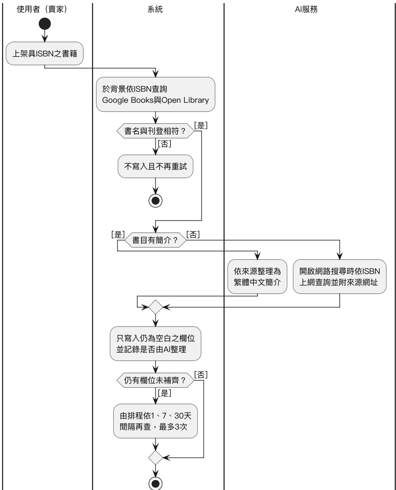
圖 5-3-29 書籍資料自動補齊之活動圖
