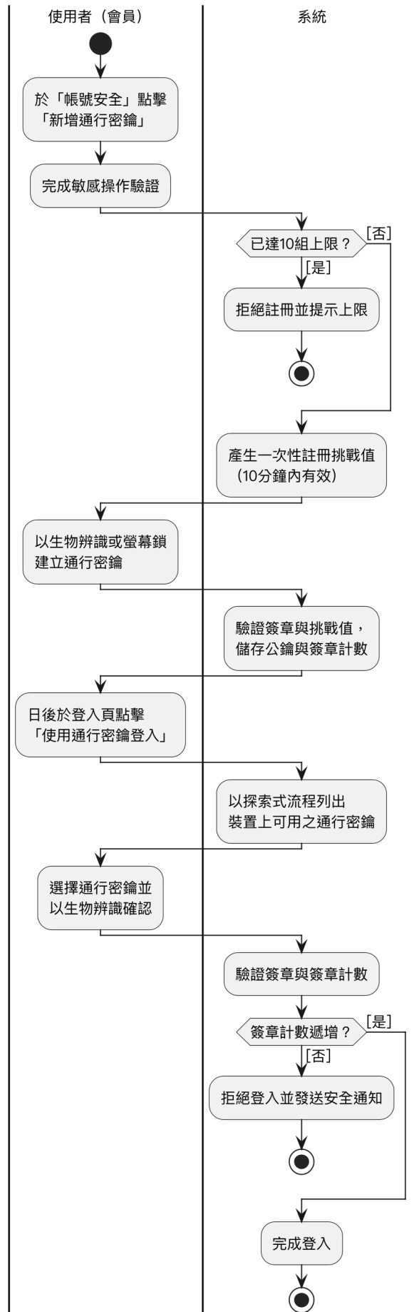
圖 5-3-14 通行密鑰 (Passkey/WebAuthn) 註冊與登入之活動圖
