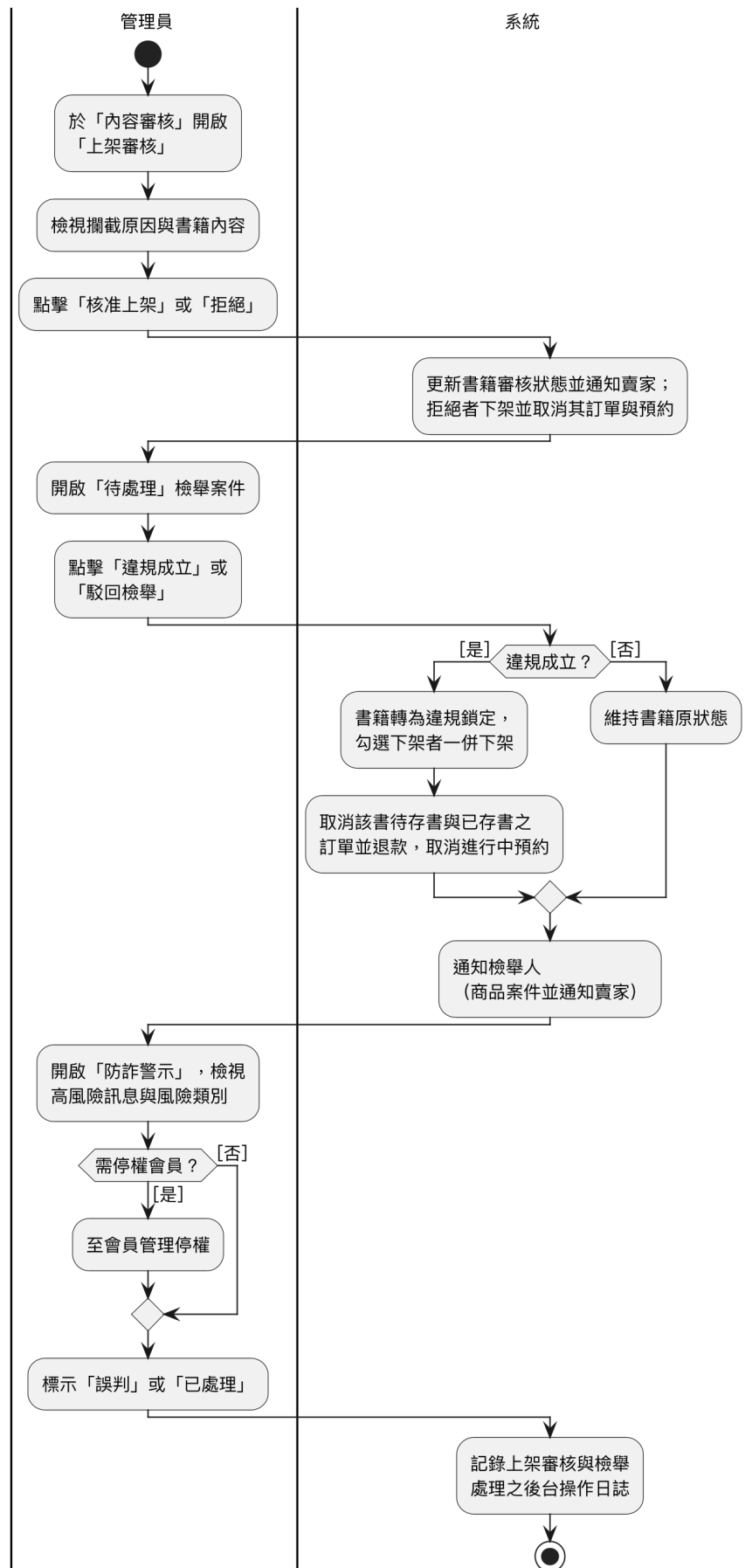
圖 5-3-11 管理員審核書籍、處理檢舉與防詐警示之活動圖
