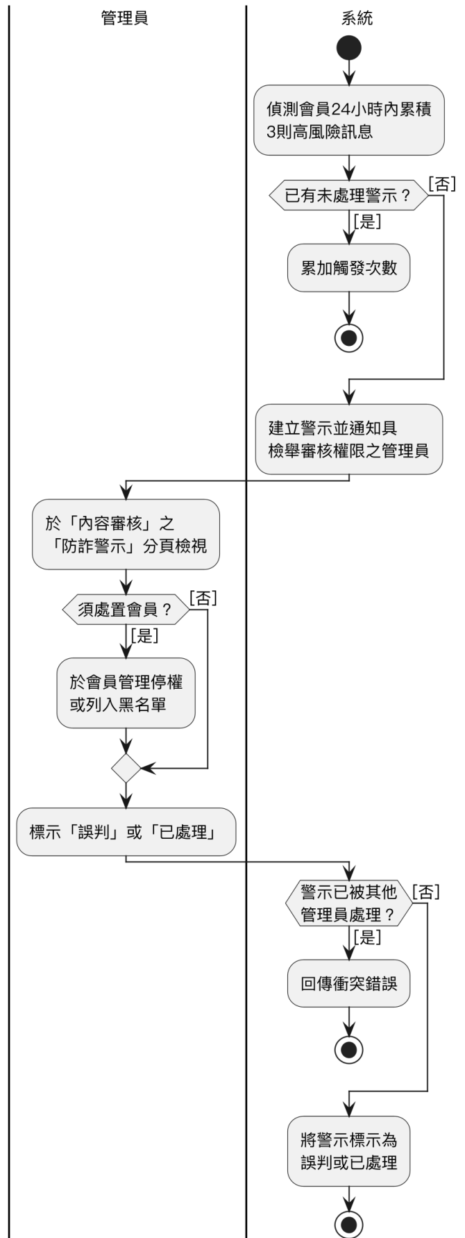
圖 5-3-30 管理員處理聊天防詐警示之活動圖
