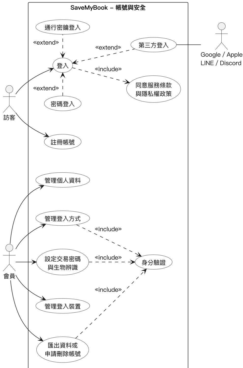
圖 5-2-1 帳號與安全模組之使用個案圖
