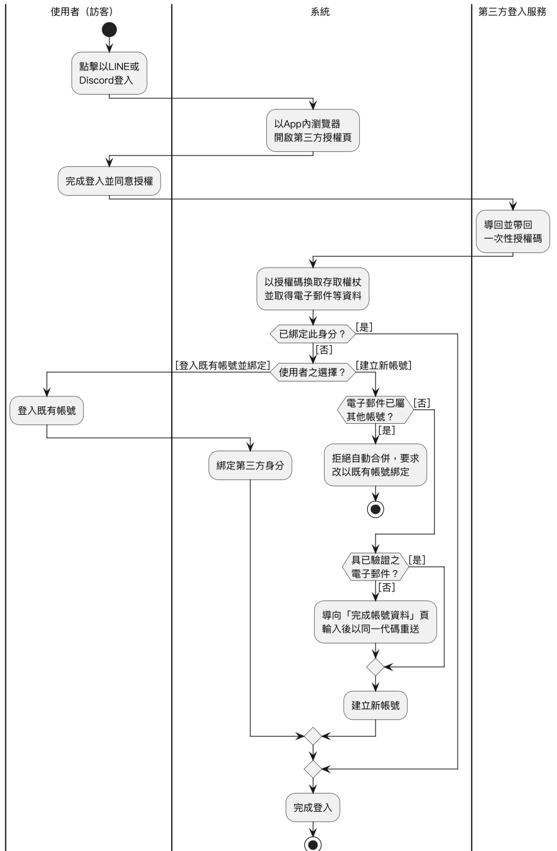
圖 5-3-26 LINE/Discord OAuth 登入與帳號連結選擇之活動圖
