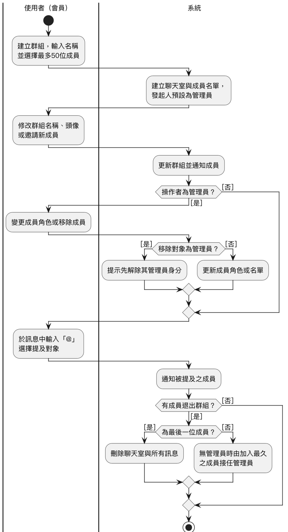
圖 5-3-19 群組聊天建立與成員管理之活動圖
