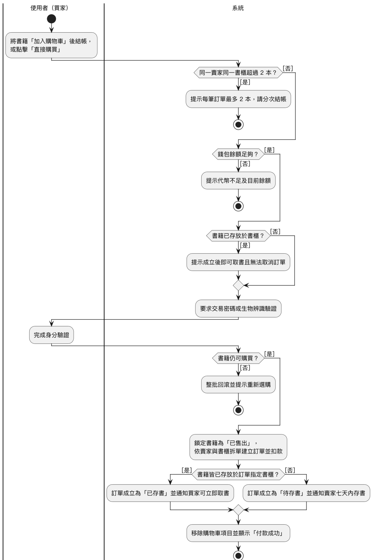
圖 5-3-4 確認訂單（加入購物車、結帳與直接購買）之活動圖
