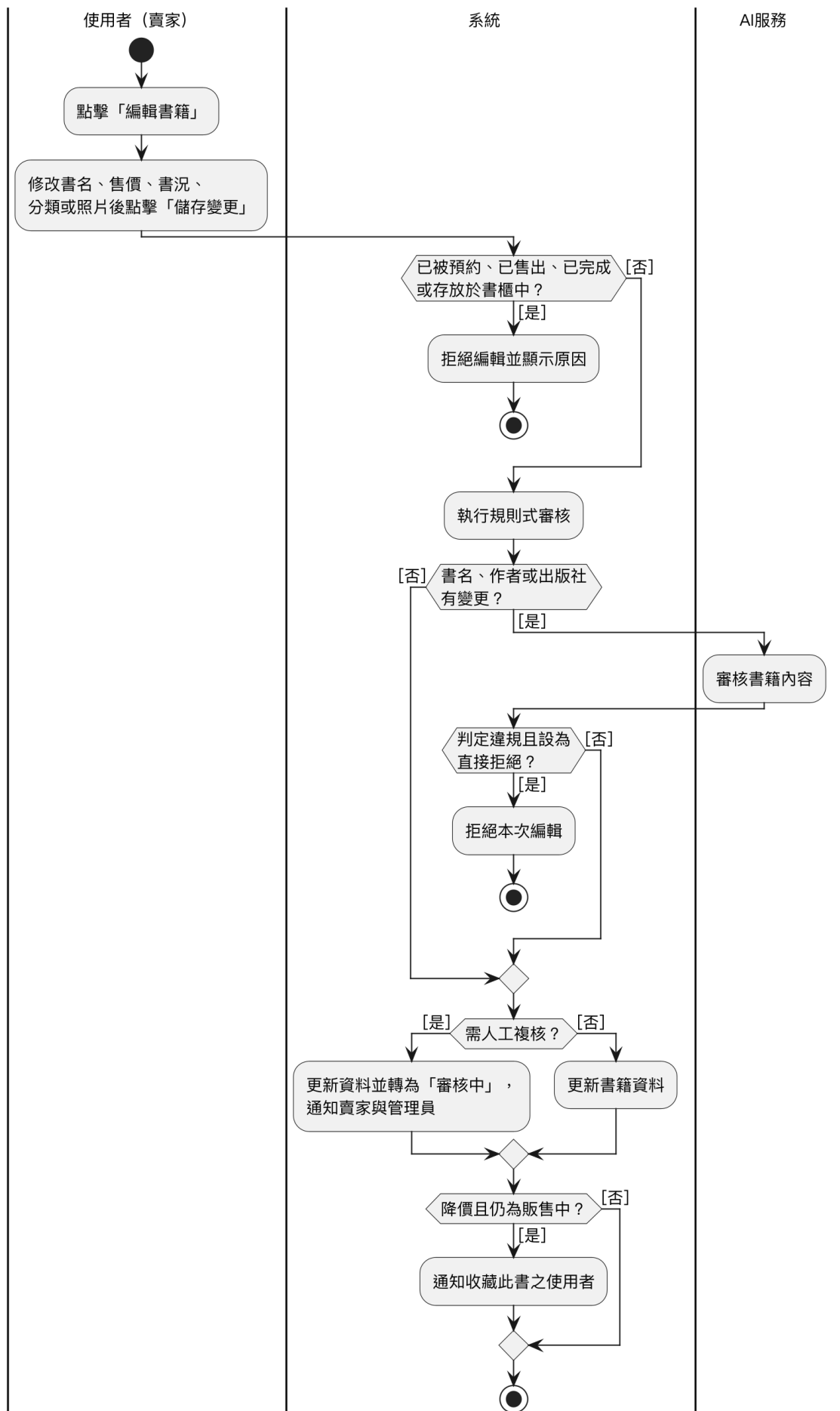
圖 5-3-2 編輯書籍之活動圖
