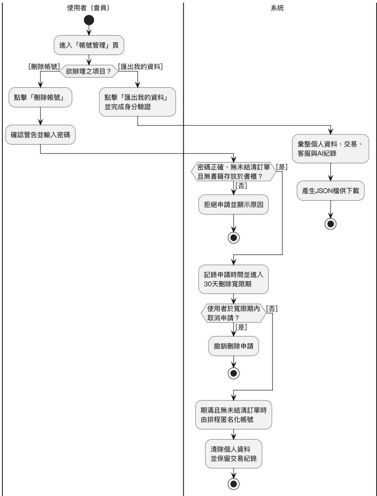
圖 5-3-17 帳號刪除申請與資料匯出之活動圖
