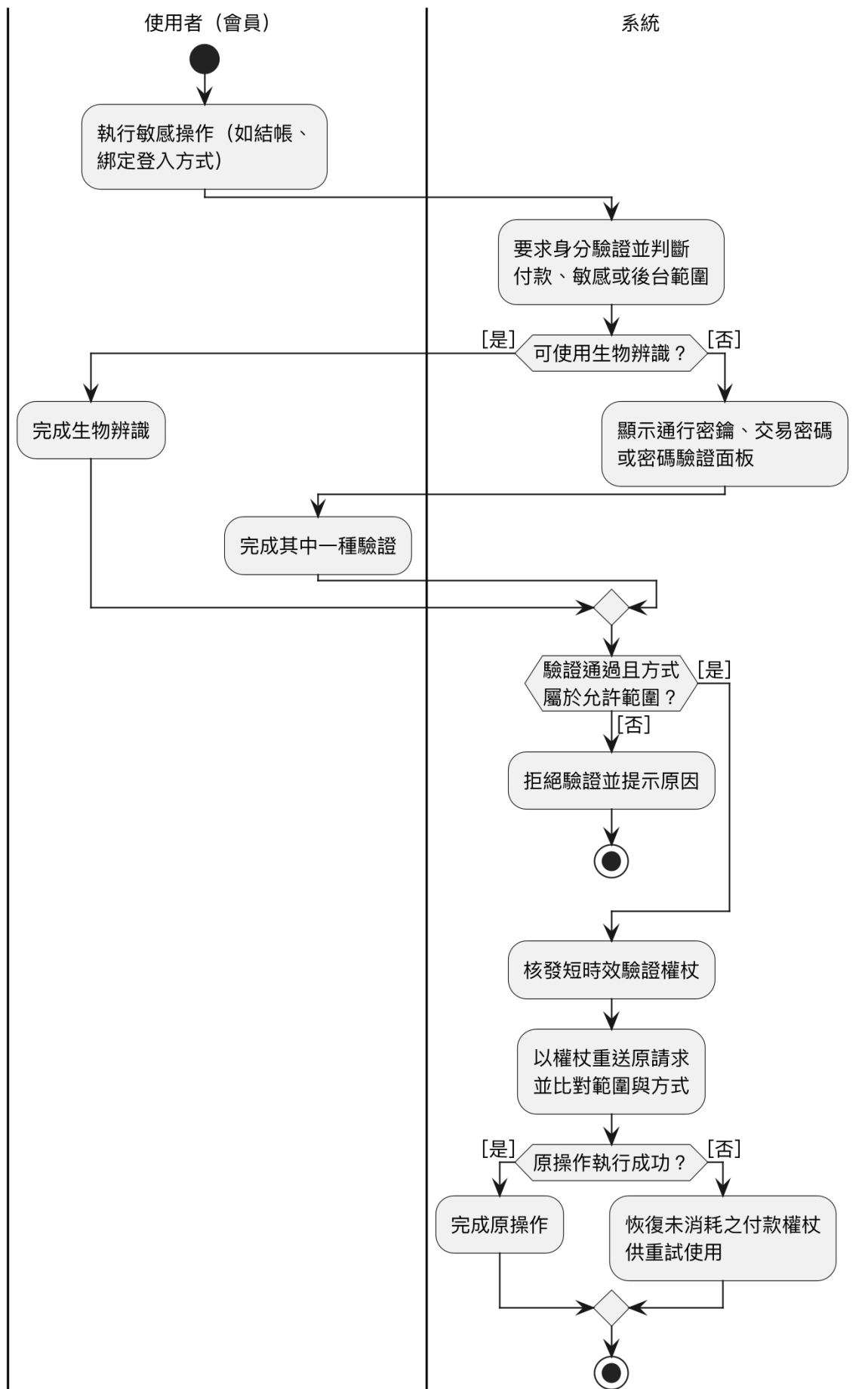
圖 5-3-15 敏感操作二次驗證之活動圖
