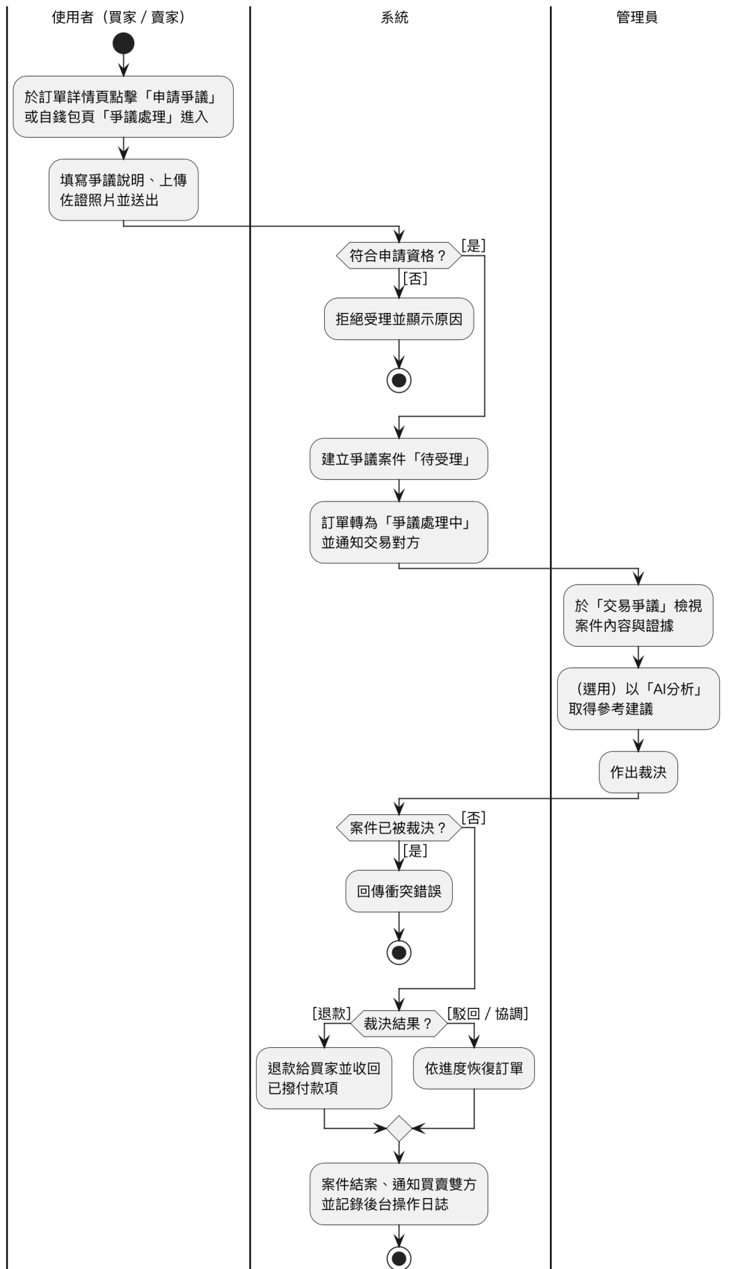
圖 5-3-7 訂單爭議與管理員裁決之活動圖
