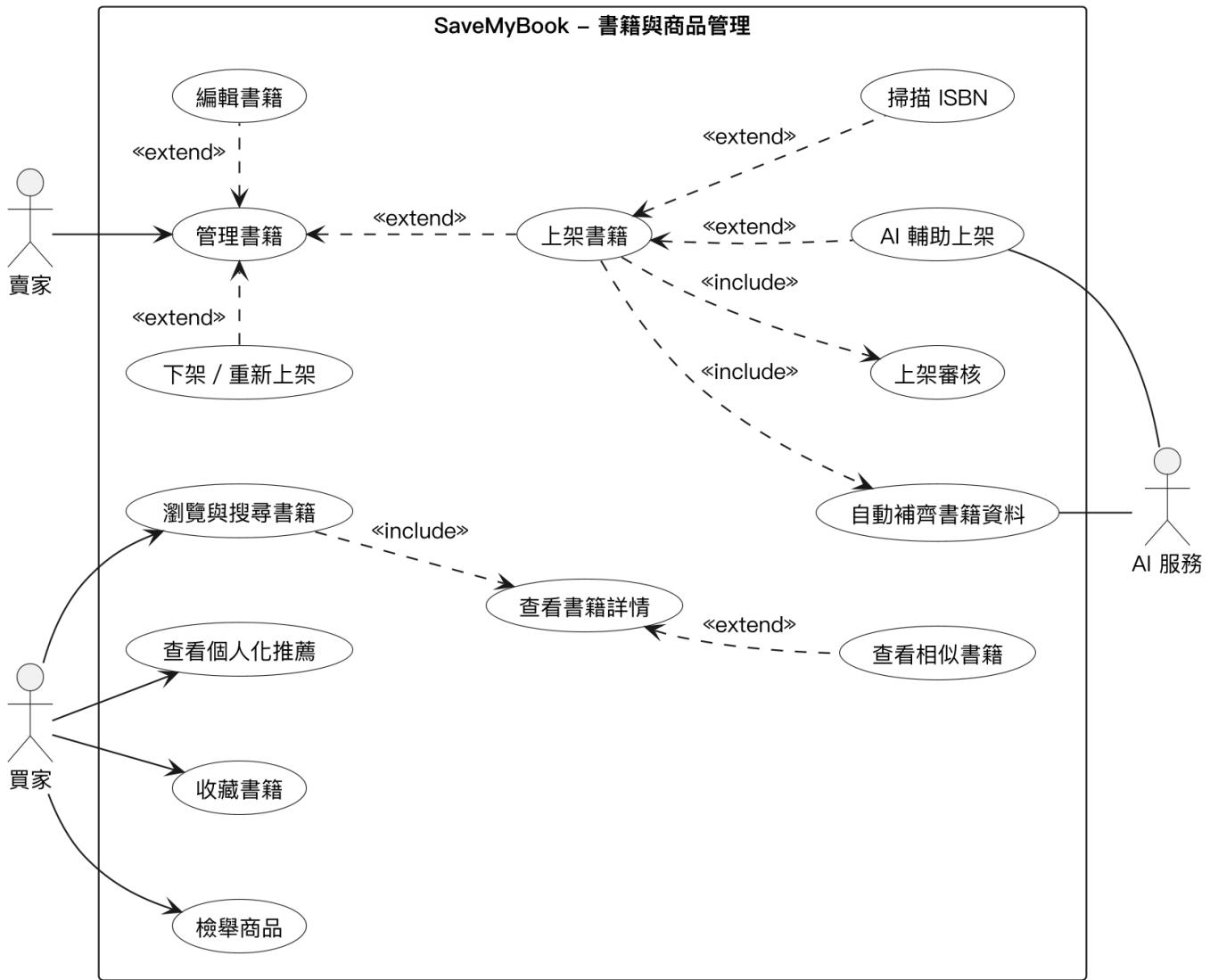
圖 5-2-2 書籍與商品管理模組之使用個案圖
