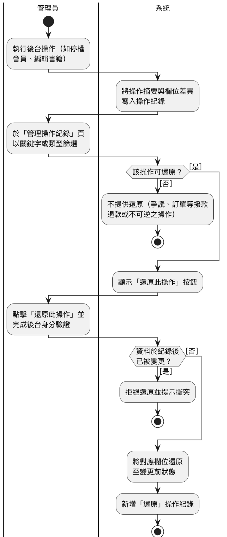
圖 5-3-21 後台操作紀錄與一鍵還原之活動圖
