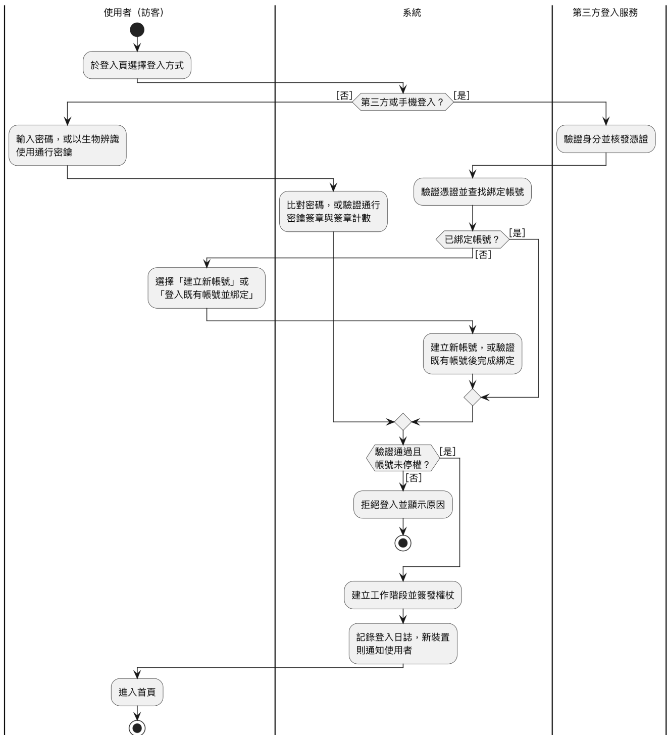
圖 5-3-8 註冊與登入（含第三方登入與 Passkey）之活動圖
