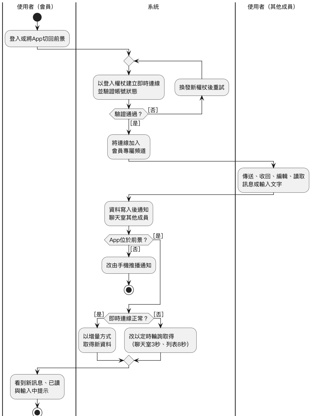
圖 5-3-28 聊天即時推送之活動圖
