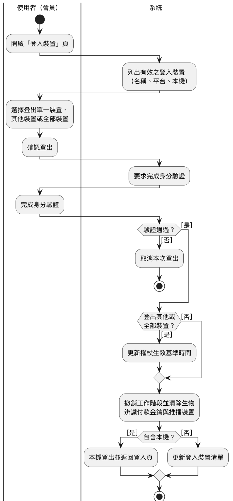
圖 5-3-16 登入裝置管理與工作階段撤銷之活動圖
