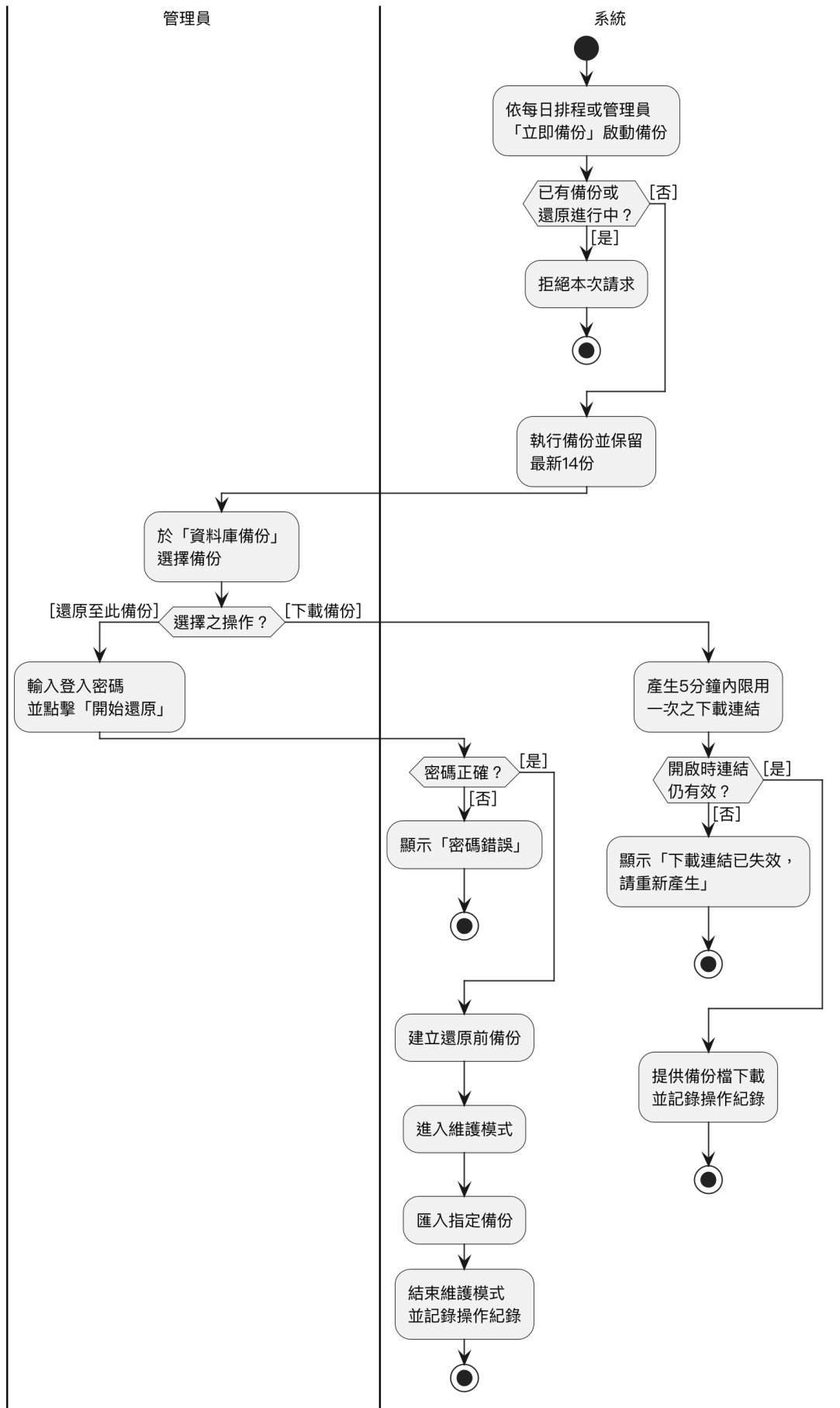
圖 5-3-22 資料庫備份與還原之活動圖
