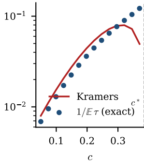
(d) escape rate
