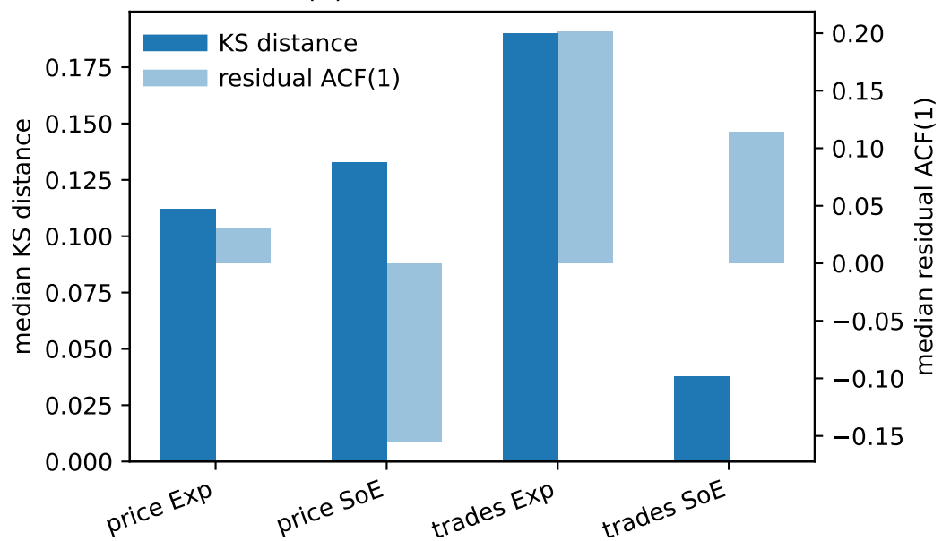
(d) residual effect sizes
