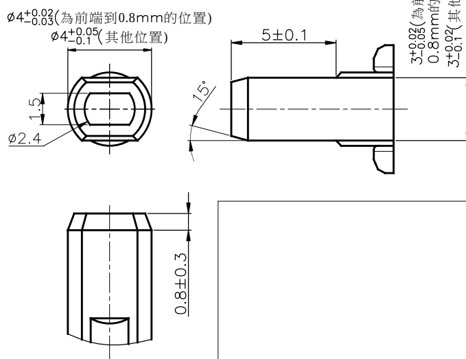
搖柄頭部尺寸(4:1)
