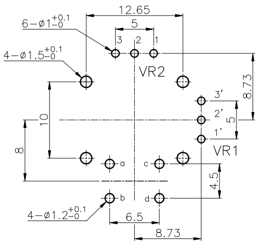
PCB板孔尺寸圖(2:1) 未注尺寸公差±0.1
