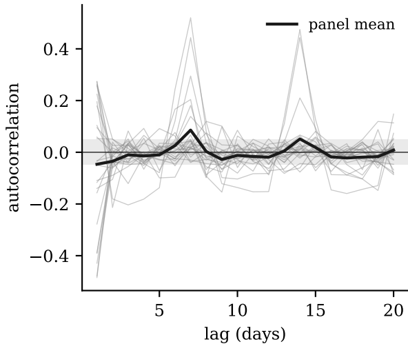
Returns r_t
