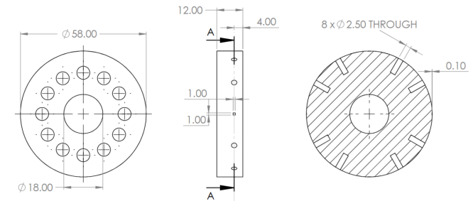
Tool flange
