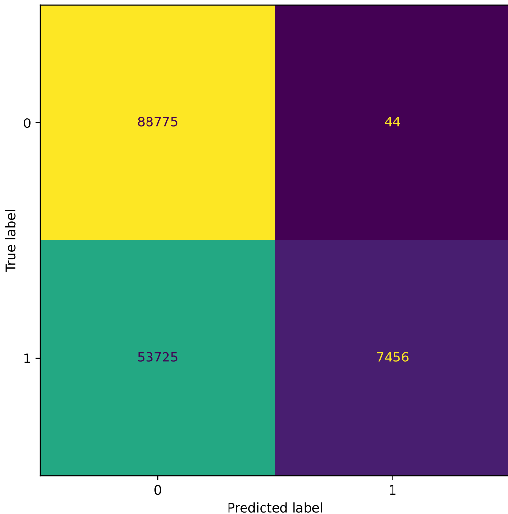
AutoEncoder
