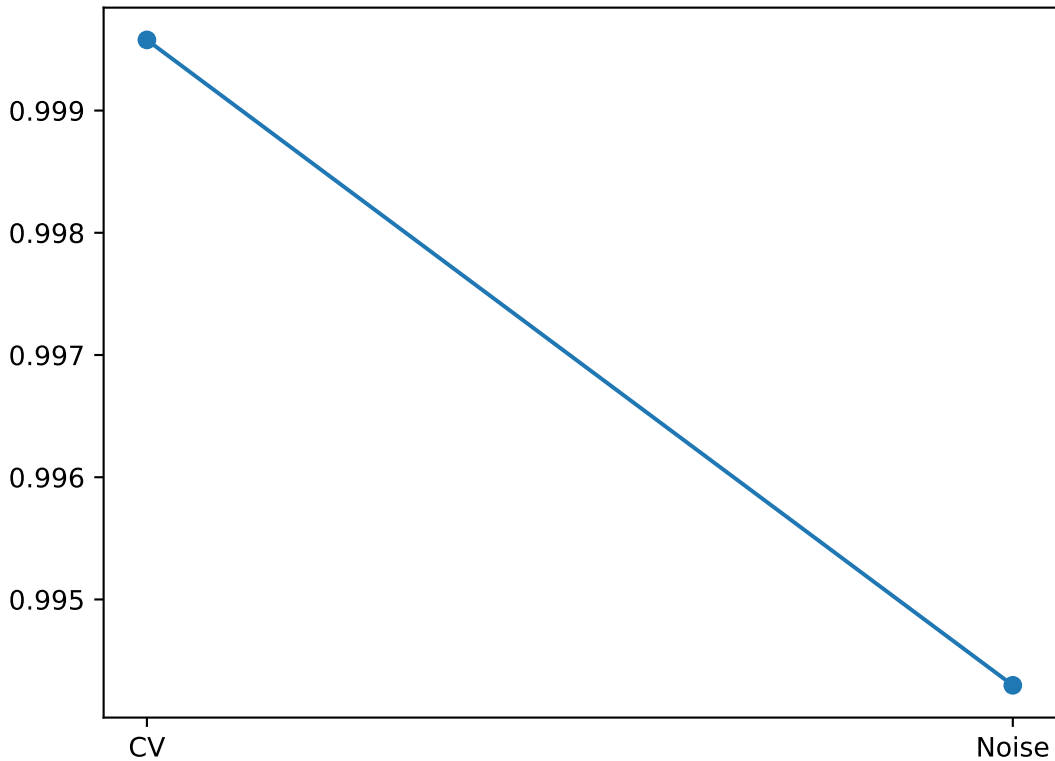
RQ6 Robustness
