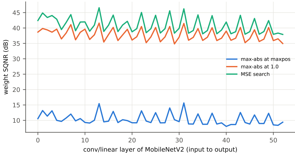
MobileNetV2, posit8_es1, per layer
