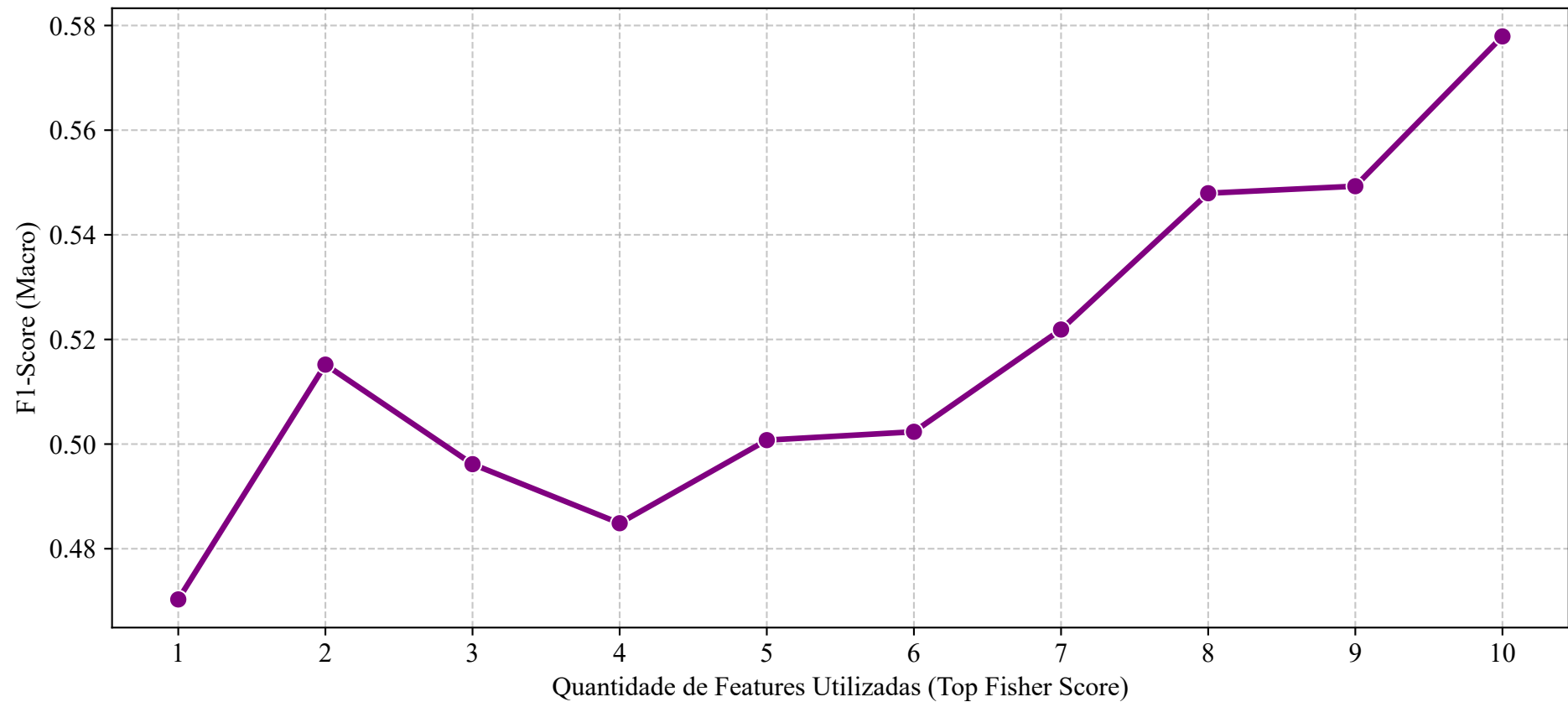
Impacto da Adição Incremental de Features Acústicas (SGD)
