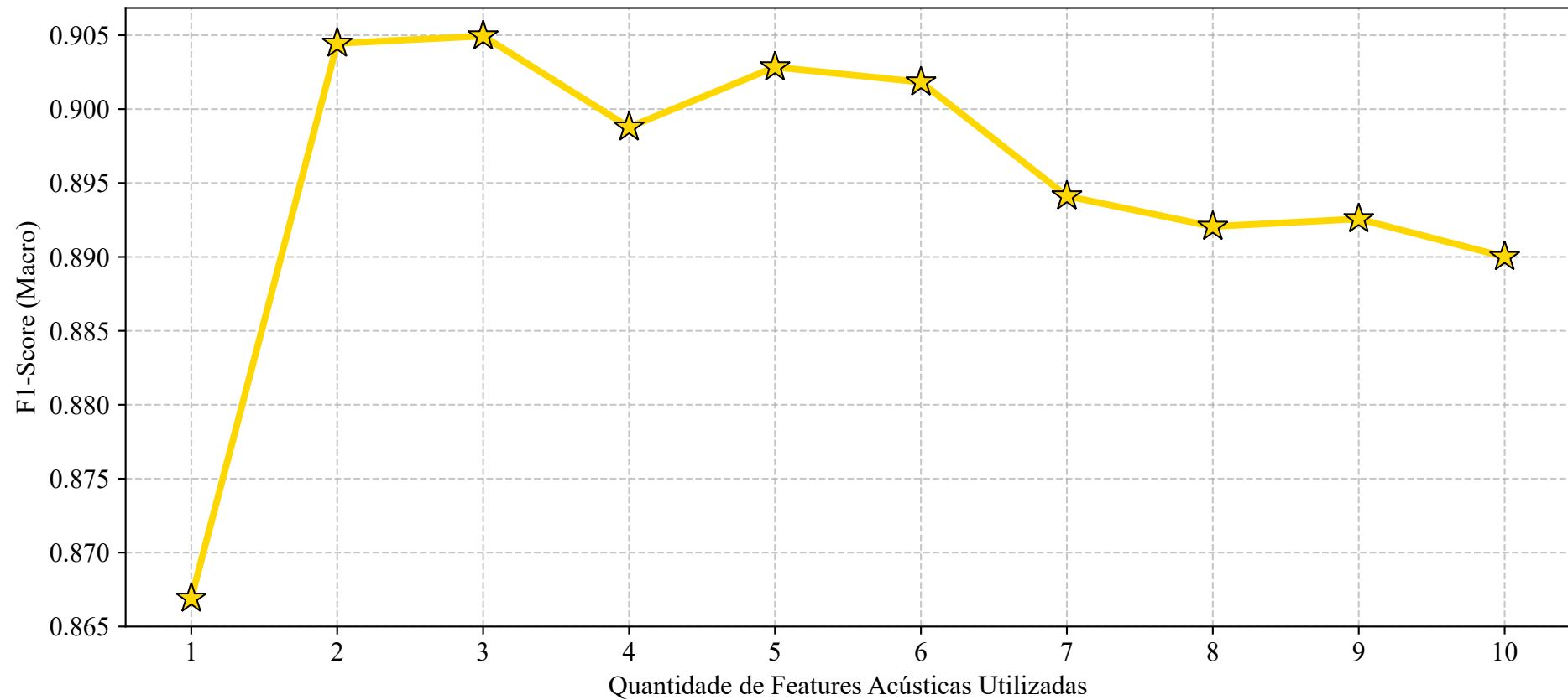
Impacto da Adição Incremental de Features no Modelo Master (NuSVC Poly Grau 3)
