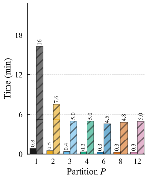
IEEE 9500-bus Time
