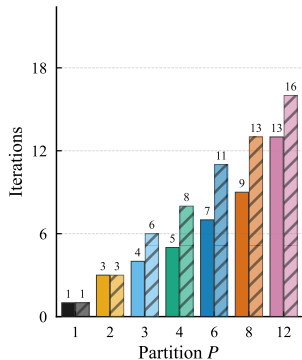
IEEE 123-bus Iterations
