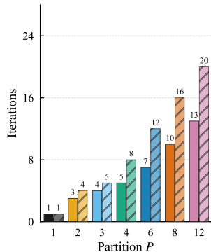
IEEE 9500-bus Iterations
