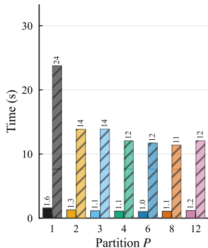
IEEE 123-bus Time
