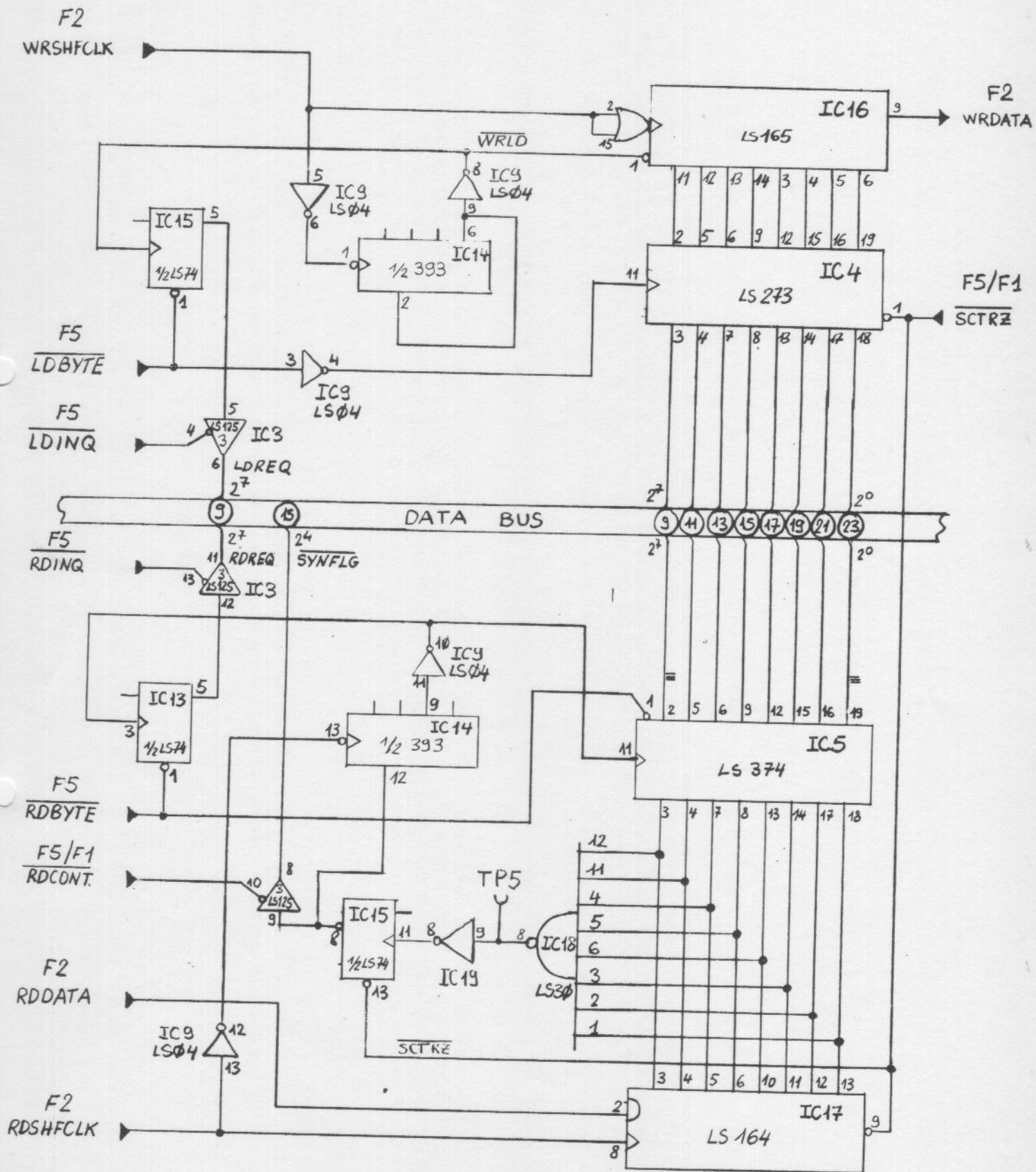
Micro-floppy contrôleur Plan F3
