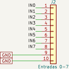
Entradas 0-7
