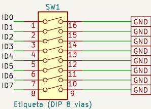
Etiqueta (DIP 8 vias)
