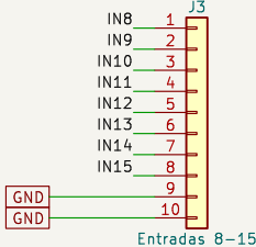
Entradas 8-15
